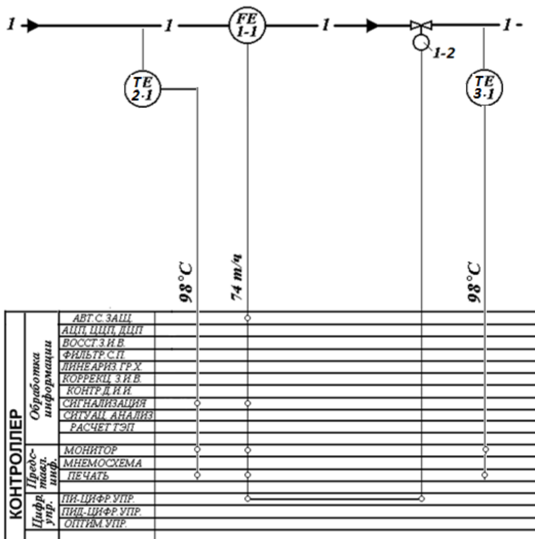
Рис.1.1. Схема автоматизации
