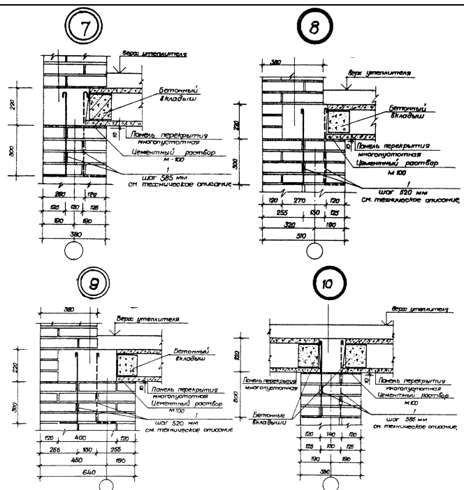
Рис. 4. Узлы анкеровки антисейсмического пояса верхнего этажа при опирании панелей перекрытий на наружные (№7, №8, №9) и внутренние (№10) стены толщиной: 380мм для узла №7; 510мм для узла №8; 640мм для узла №9; 380мм для узла №10
