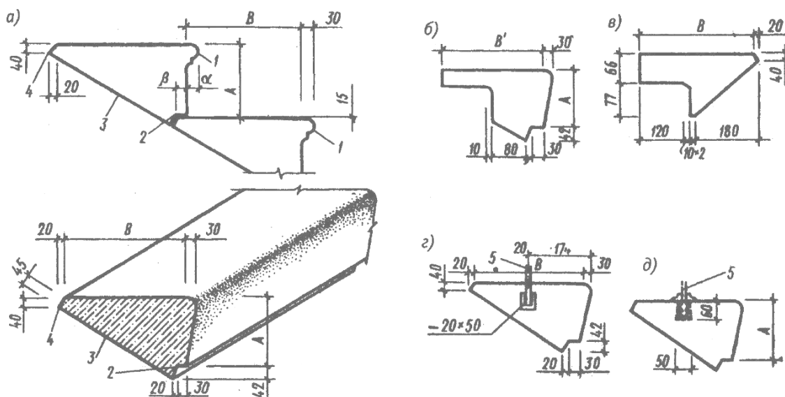
Рис. 40. Конструктивные виды внутренних сборных железобетонных мелкоэлементных лестничных ступеней: а-рядовые ступени; б-верхняя фризная ступень; в-нижняя фризная ступень; г-крепление стойки ограждения лестничного марша к боковой поверхности ступени; д-то же, к верхней поверхности ступени; 1-валик; 2-хвост; 3-постель; 4-замок; 5-стойка ограждения лестничного марша
