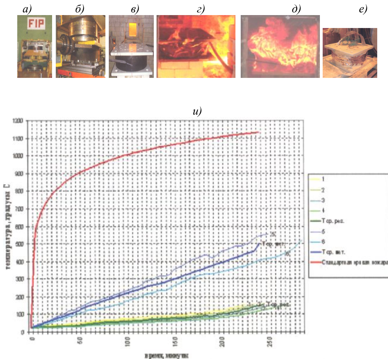
Рис. 87. Натурные испытания сейсмоизолирующих резинометаллических опор на специальном оборудовании в лабораторных условиях: а, б -испытания сейсмоизолирующих резинометаллических опор (СРО) на прочность под гидравлическим прессом; в, г, д –испытания СРО с огнезащитным покрытием «Термал» по огнестойкости в специальной печи; е –то же, после испытания на огнестойкость; и –график зависимости температуры в печи с образцом СРО, t^{\circ}\text{C} от времени T , в минутах t=f(T) для разных типов огнезащитных покрытий
