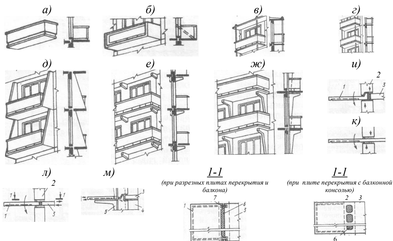
Рис. 47. Примеры конструктивных решений балконов:
