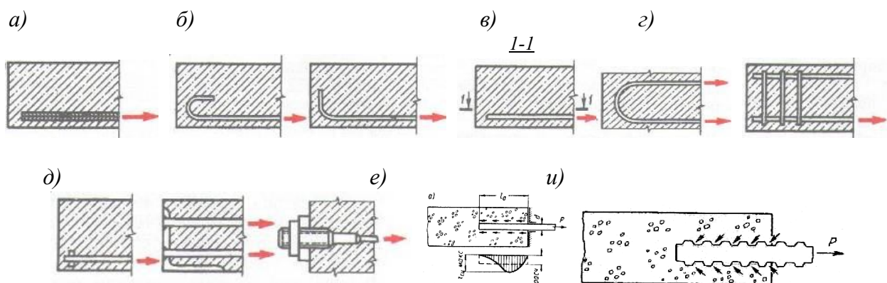
Рис. 53. Анкерование арматуры в бетон:
