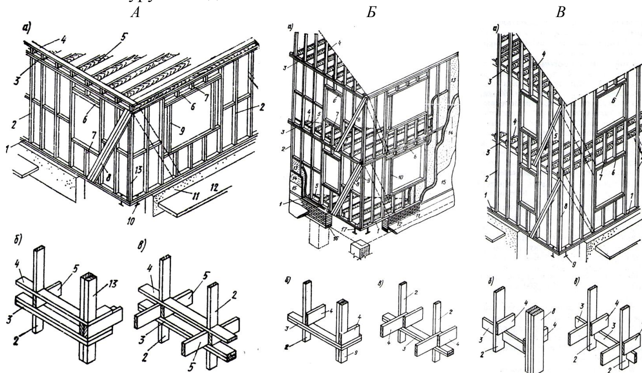
Рис. 73. Конструкции каркасного дома: А -с платформенным сопряжением стоек; Б -с контактным сопряжением стоек; В -с засыпным каркасом; а -общий вид каркаса; б -опирание балок на наружную стену в углу; в -опирание балок на внутреннюю стену; 1-нижняя обвязка; 2-стойка 50x100мм, 50x150мм; 3-верхняя обвязка 2(50x100мм)- для А , Б и опорная доска на ребро 50x150мм- В ; 4-вторая обвязка 50x100мм-для А , балка перекрытия 50x200мм-для Б , В ; 5-балка перекрытия 50x200мм-для А , распорка 50x200мм-для Б , раскосы жесткости -для В ; 6-балка-перемычка-для А , Б и В ; 7-укороченная стойка; 8-раскосы жесткости -для А и Б , доборные стойки в углах 50x150мм -для В ; 9-дополнительная стойка проема -для А , доборные стойки в углах 50x100мм -для Б ; 10-анкерные болты -для А , дополнительная стойка проёма -для Б ; 11-цоколь; 12-отмостка; 13-доборные стойки в углах 50x100мм -для А , утеплитель между стойками -для Б ; 14-утеплитель снаружи -для Б ; 15-штукатурка -для Б ; 16-фундаментная балка -для Б ; 17-анкерные болты -для Б
