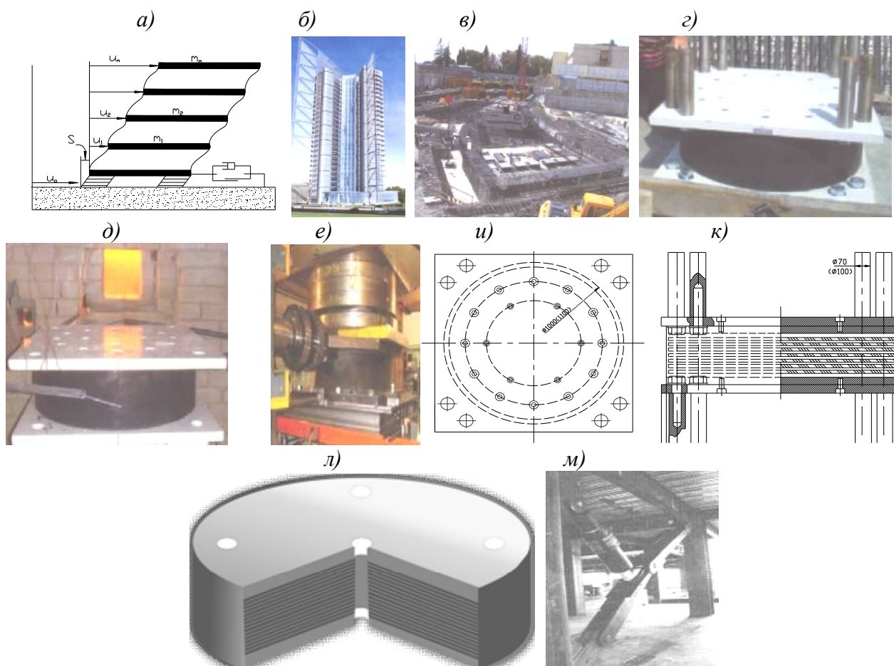
Рис. 18. Система пассивной и активной сейсмоизоляции зданий и сооружений: а-модель системы «сооружение-сейсмоизолирующий фундамент-грунт»; б-фасад сейсмоизолированного гостинично-туристического комплекса «Sea Plaza» в г. Сочи; в-возведение сейсмоизолированного фундамента; г-сейсмоизолирующая опора перед монтажом фундамента (пассивная сейсмоизоляция); д, е-испытание сейсмоизолирующей опоры огнем и под прессом «RIG 80» фирмы «FIP Industriale S.p.A» (Италия); и, к, л-план, разрез и общий вид резинометаллической опоры с высокодемпфирующей резиной типов SI-H 1000/168; м- сейсмозащита здания «Башня Yerba Buena» в Сан-Франциско, с диагоналями и жидкостными демпферами (активная сейсмоизоляция)
