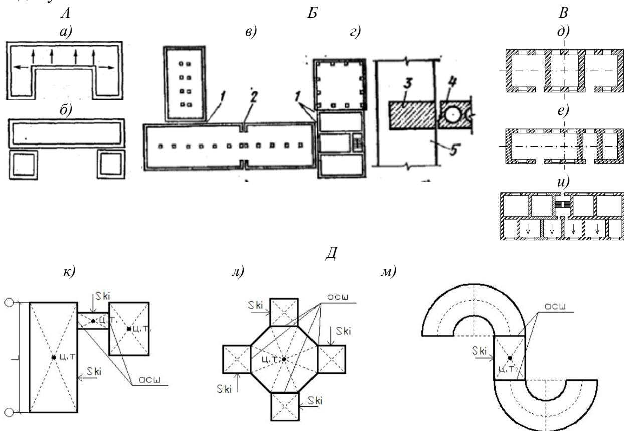
Рис. 25. Антисейсмические мероприятия и принципиальные схемы вариантов сложных геометрических форм зданий или сооружений в плане, и наиболее опасные направления действия сейсмических воздействий S_{ki} :
