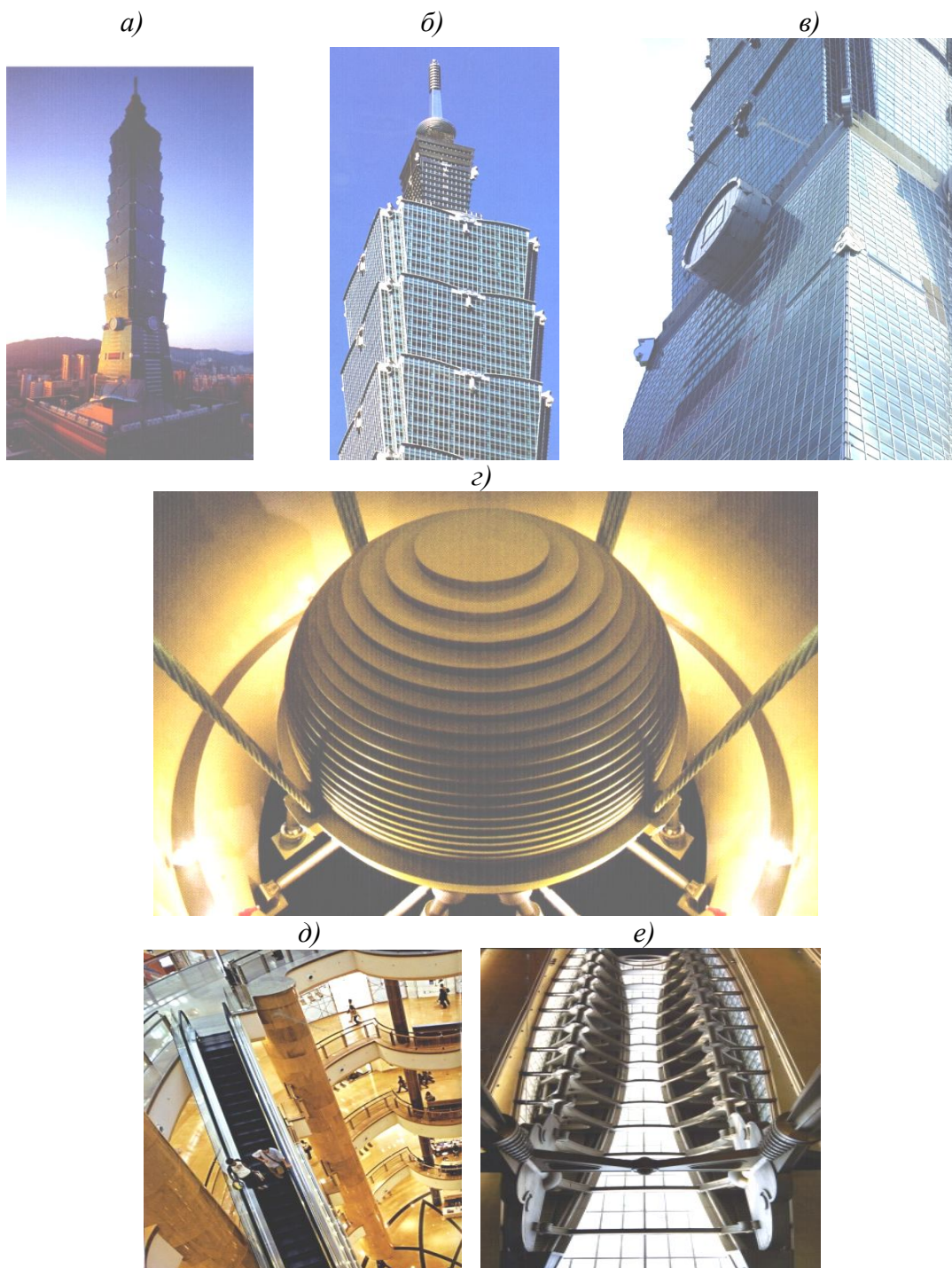
Рис. 3. Практическое использование инерционной массы, выполняющей функцию «гасителя» сейсмического колебания во время землетрясения на примере 101-этажного небоскреба Тайбэй-101, высотой 1671 фут или 509 метров, возведенного в 2004 году по проекту архитектора китайского происхождения Чан-Юн-Ли, расположенного в столице Тайваня - городе Тайбэй в Китайской Республике:
