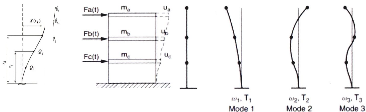
Рис. 83. Схема консольной расчетной динамической модели
