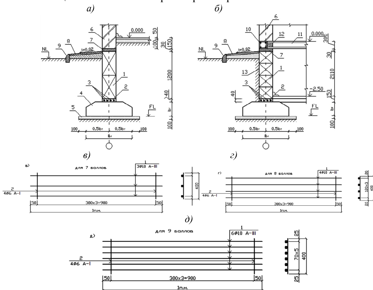
Рис. 30. Конструктивные решения по обеспечению расчетной сейсмостойкости подземной части стен и фундаментов, возводимых из сборных бетонных и железобетонных конструкций для зданий без подвала (а) и с подвалом (б):
