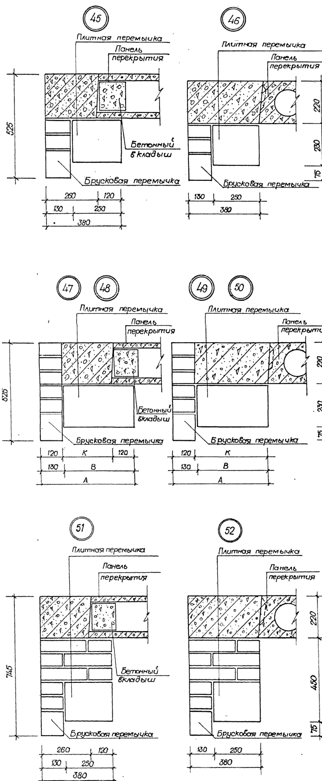
Рис. 8. Узлы №35 - №52. Комплексные конструкции. Примеры сечений железобетонных перемычек в стенах толщиной 380, 510 и 640 мм, при высоте этажа 2,80м и 3,00м
