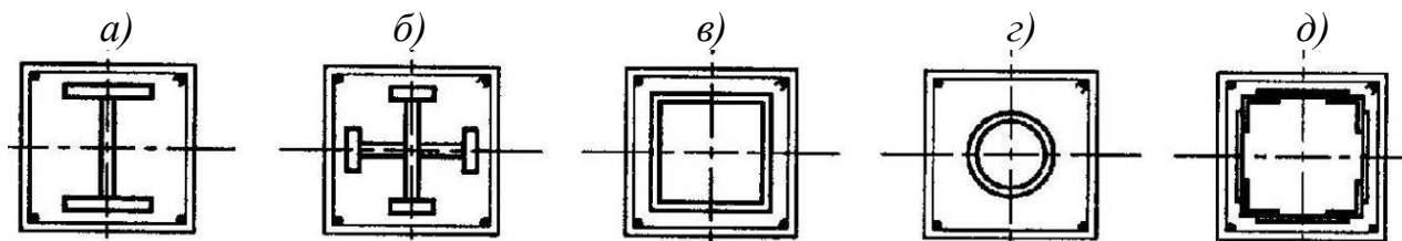
Рис. 56. Типы поперечных сечений сталежелезобетонных колонн нижних «гибких» этажей с жесткой арматурой из различных стальных профилей
