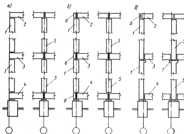
Рис. 80. Варианты привязки наружных и внутренних несущих панельных стен к координационным осям: а, б – платформенный вариант опирания; в – контактный стык панелей; 1-наружная панель; 2-чердачное перекрытие; 3-междуэтажное перекрытие; 4-цокольное перекрытие; 5-внутренняя панель; 6-доборная обвязка; 7-опорный брус
