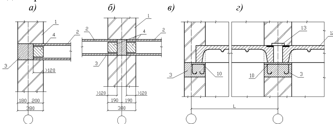
Рис. 72. Узлы опирания многопустотных и ребристых плит перекрытий и покрытия на кирпичные стены с устройством системы горизонтальных дисков жесткости при помощи устройства сейсмических поясов: а-опирание многопустотной плиты на крайнюю стену; б-то же, на среднюю стену; 1-кирпичная стена; 2-многопустотная железобетонная плита; 3-сейсмопояс по типовой серии 2.140-5с; 4-бетонный вкладыш в пустотах; в-опирание ребристой плиты на крайнюю стену; г-то же, на среднюю стену; 3-сейсмопояс по типовой серии 2.140-5с; 10-закладная деталь в теле сейсмопояса; 12-сборная железобетонная ребристая плита перекрытия; 13-накладная деталь, привариваемая к закладным деталям в плитах перекрытий
