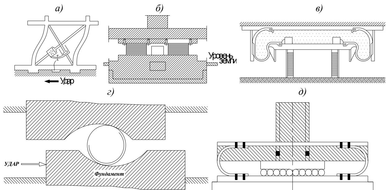
Рис. 13. Современные системы сейсмозащиты и сейсмоизоляции зданий и сооружений: а-схема устройства для изменения жесткостных характеристик здания и его динамических параметров; б-резинометаллический сейсмоизолятор; в-сейсмоизолятор с воздушной подушкой высокого давления; г-сейсмоизолятор со скользящими поясами с использованием эффекта трения-скольжения
