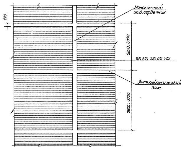
Рис. 3. Фрагмент фронтальной проекции кирпичной кладки стены с одиночным железобетонным включением комплексной конструкции
