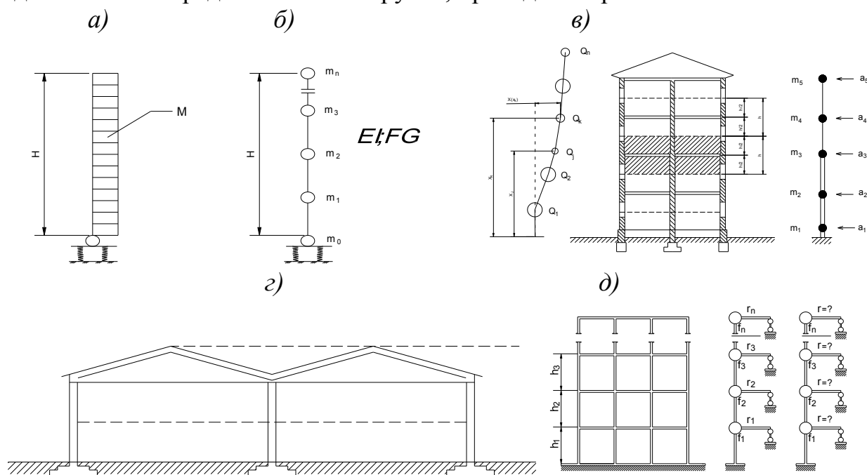
Рис. 21. Расчетные и конструктивные схемы одноэтажных и многоэтажных кирпичных и каркасных зданий, возводимых в сейсмических районах:
