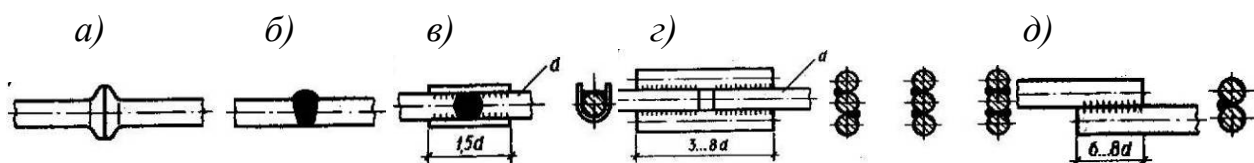
Рис. 52. Основные типы сварных соединений арматуры:
