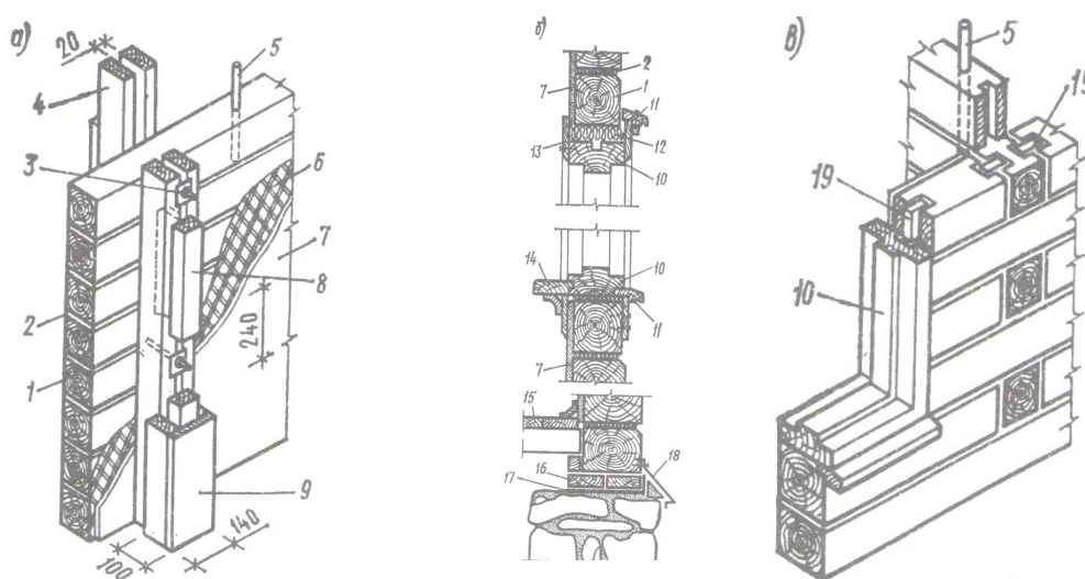
Рис. 77. Конструктивные решения в брусчатых стенах: а-устройство сжима в брусчатой стене; б-узлы разрезов по окну и цоколю; в-сопряжение стен и установка оконной коробки; 1- брус; 2-конопатка; 3-натяжной болт-костыль M12 , l=400 мм через 4 венца; 4-сжимы 2 (50x100мм); 5-нагель; 6- дранка; 7- штукатурка; 8-бобышка 50x80x400мм с прокладками 20x100x400мм; 9-наличник из досок \delta=20 мм; 10-оконная коробка; 11-наличник оконный наружный; 12-зазор 1/20 от высоты проема; 13-наличник оконный внутренний; 14-подоконник; 15-чистый пол; 16-антисептированная прокладка; 17-гидроизоляция (два слоя рубероида); 18-отлив из стали; 19-шип
