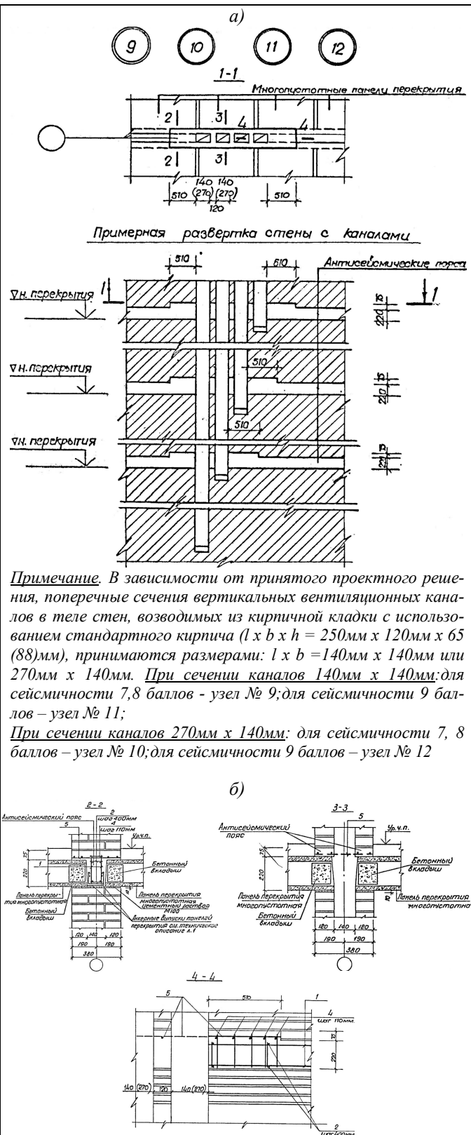
Рис. 4. Узлы № 9, 10, 11, 12 опирания сборных многопустотных панелей перекрытий на средние (внутренние) несущие кирпичные стены с вертикальными каналами для вентиляции и дымоудаления: а – фрагмент плана и разрез 1-1; б – сечения 2-2, 3-3, 4-4 к узлам № 9, 10, 11, 12
