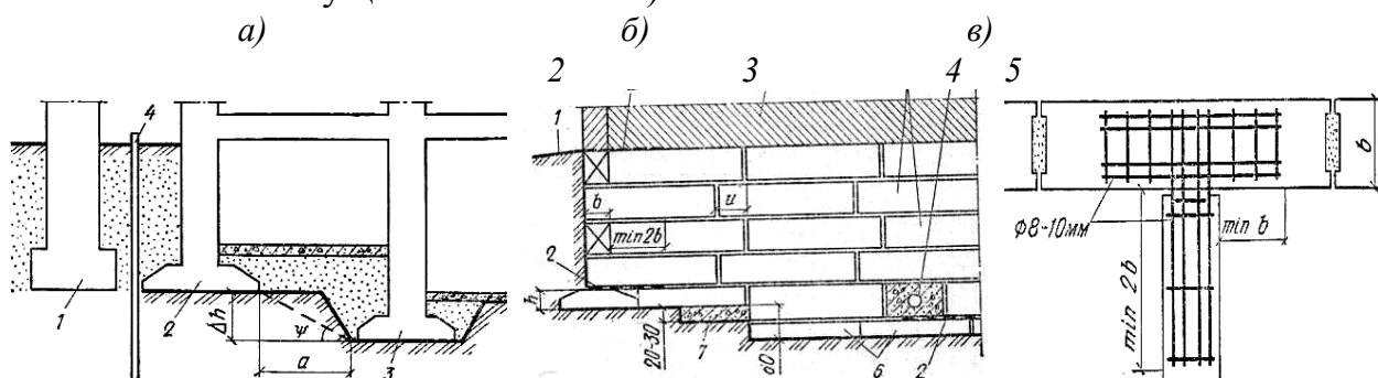
Рис. 29. Расчетно-конструктивные схемы к инженерным мероприятиям по размещению отметки подошвы фундаментов на разных уровнях:
