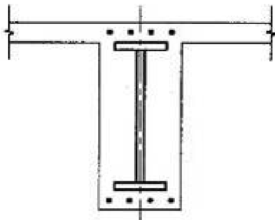
Рис. 58. Поперечное сечение железобетонной балки с жесткой арматурой из стальных профилей
