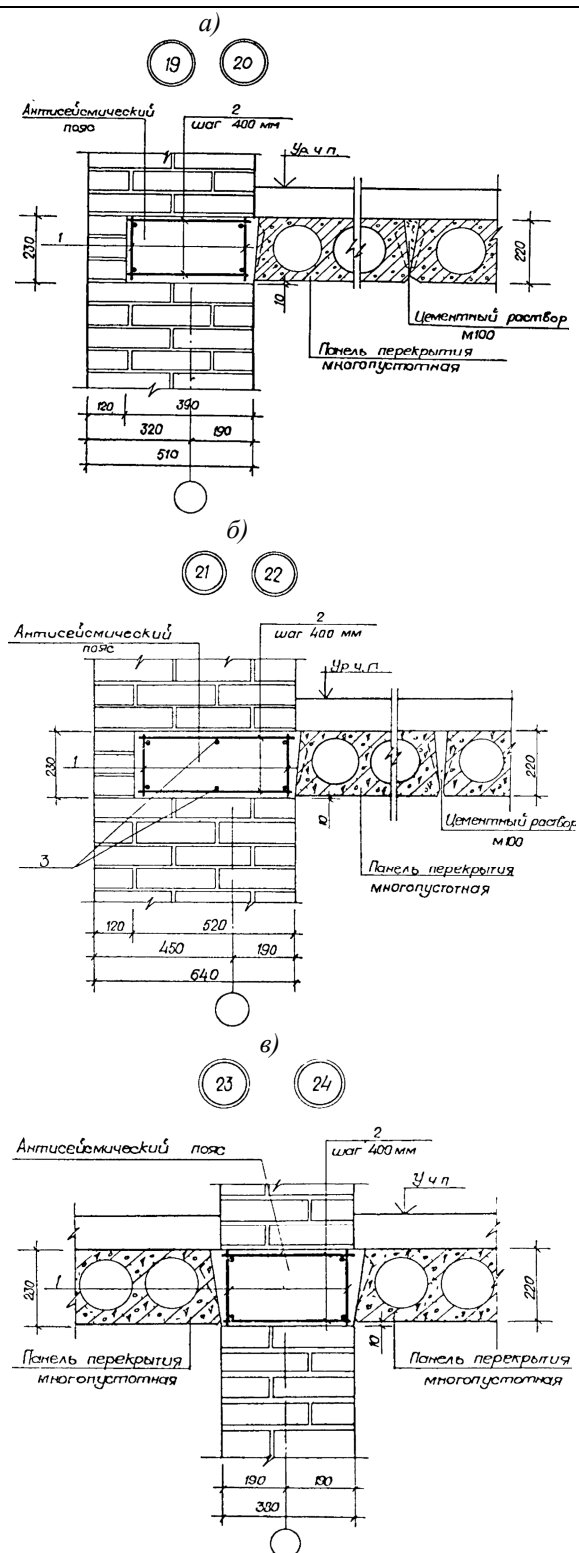
Рис. 8. Узлы № 19, 20, 21, 22, для наружных стен и № 23, 24 для внутренних стен с примыканием сборных многослойных панелей перекрытий к самонесущим кирпичным стенам: а - № 19, 20 для наружных стен толщиной 510мм, где № 19-для 7, 8 баллов, №20-для 9 баллов; б - № 21, 22 для наружных стен толщиной 640мм, где № 21-для 7, 8 баллов, № 22-для 9 баллов; в - № 23, 24 для внутренних стен толщиной 380мм, где №23-для 7, 8 баллов, № 24-для 9 баллов
