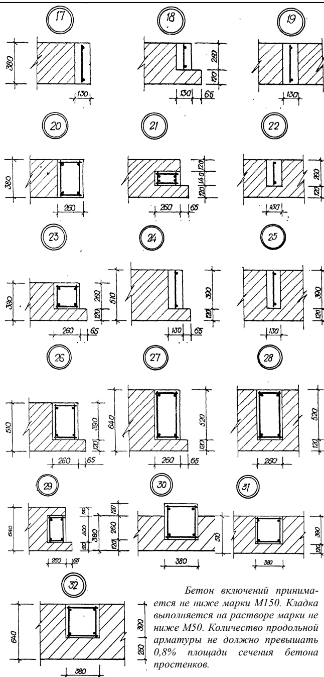
Рис. 6. Узлы №17 - №32. Комплексные конструкции. Примеры сечений железобетонных включений в стенах толщиной 380, 510 и 640 мм
