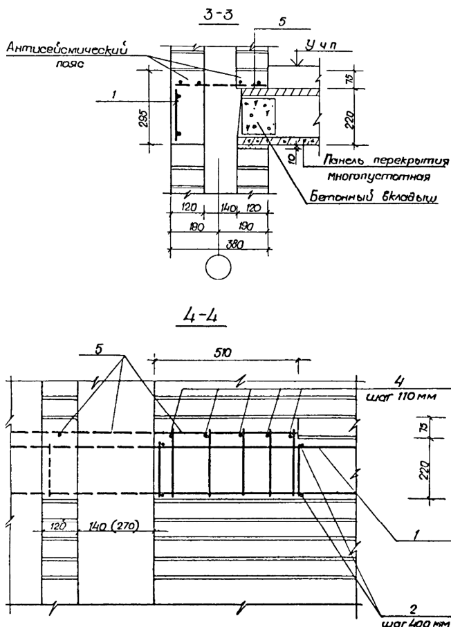
Рис. 6. Сечения 3-3 и 4-4 к узлам № 13, 14, 15, 16 на рис. 5 опирания сборных многпустотных панелей перекрытий на крайние несущие кирпичные стены с вертикальными каналами для вентиляции и дымоудаления
