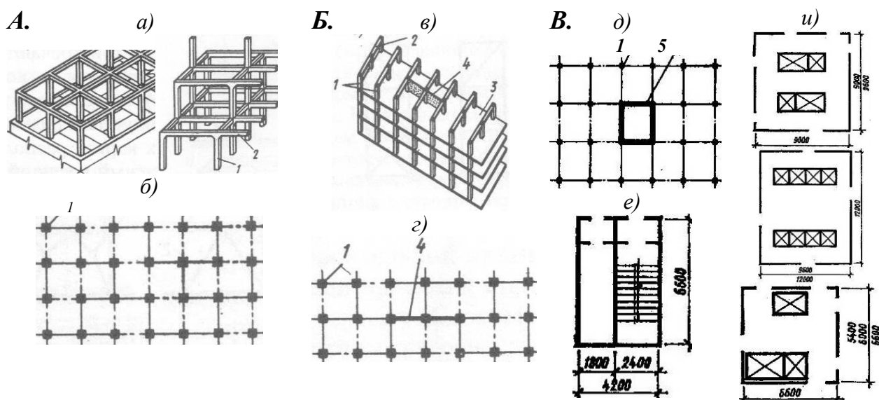
Рис. 54. Конструктивные схемы каркасных остовов:
