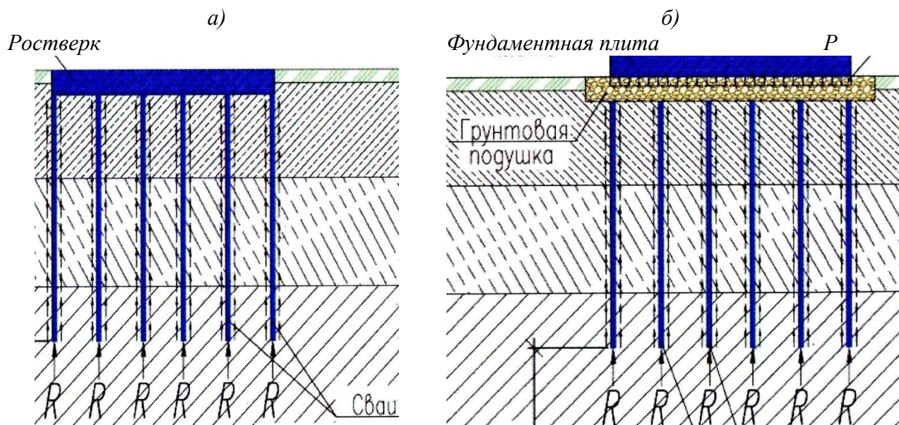
Рис. 34. Принципиальные схемы (КСПФ) комбинированного свайно-плитного фундамента (а); и сплошного плитного фундамента, возведенного на вертикально армированном грунтовом основании с демпфирующей грунтовой подушкой (б); P —среднее давление под фундаментом; R —расчетное сопротивление грунта под свайей или вертикальным армоэлементом
