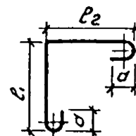
Рис. 18. Отдельные арматурные стержни OC-7, OC-8 по ГОСТ 5781-82
