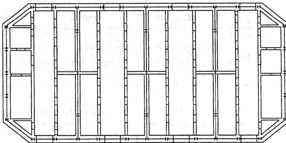
Рис. 57. План расположения элементов жесткого армирования из стальных профилей в стенах ствола ядра жесткости, выполненного из монолитного железобетона
