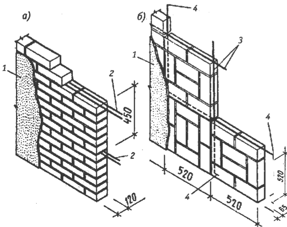
Рис. 44. Конструкции мелкоштучных перегородок для сейсмических районов: а - армокирпичная толщиной 120 мм (1/2 кирпича); б - то же, 65 мм (1/4 кирпича); 1 - отделочный слой; 2 - арматура d=3...6 мм для горизонтального армирования перегородки в ее кладочных швах; 3 - то же, вертикального армирования d=4...6 мм; 4 - отгибы арматуры для крепления к стенам и перекрытию
