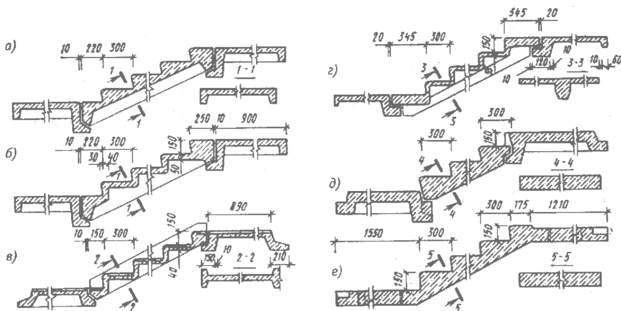
Рис. 41. Конструктивные решения внутренних полносборных железобетонных лестниц: а – с - П-образными ребристыми маршами; б – с - П-образными складчатыми маршами; в – с - Н-образными складчатыми маршами; г – с - Т-образными складчатыми маршами; д - марши плитной конструкции; е - марши плитной конструкции, совмещенные с полуплощад- ками (Z-образной формы)
