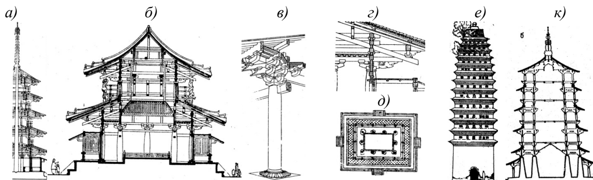
Рис. 11. Сейсмостойкие конструкции и тектонические особенности зданий и сооружений в архитектуре Японии и Китая: а-фрагмент разреза сооружения монастыря Хорюдзи в Нара (Япония), VII в.; б-поперечный разрез кондо; в-ордер с системой «доугун»; г-конструкция опирания крыши на стойки; д-план конда; е-фасад кирпичной пагоды Цзючжобуа в провинции Сычуань (Китай) 1000 г; ж-разрез по пагоде в провинции Шаньси (Китай) 1056 г
