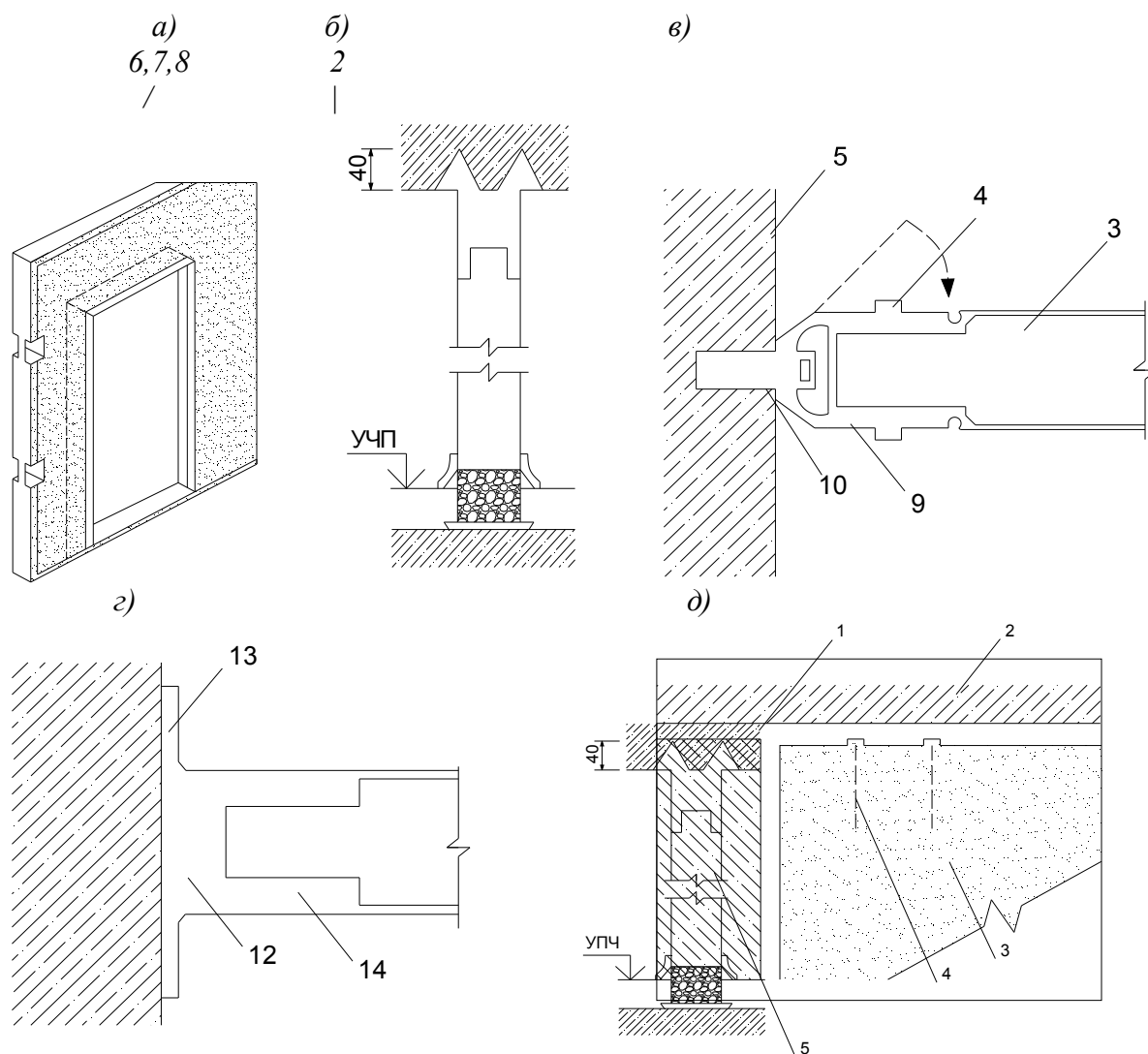
Рис. 45. Облегченные крупнопанельные гипсолитовые перегородки: а -общий вид; б -узел крепления перегородки кверху и низу перекрытия; в , г - крепление боковых сторон перегородки к стенам (перегородкам); д -податливое крепление верхнего уровня перегородки к перекрытию; 1-металлический анкер из полосы 4х25 мм; 2-железобетонная плита перекрытия; 3-перегородка; 4- гвоздь (шуруп); 5-стена (перегородка); 6, 7, 8-деревянная обвязка перегородки; 9-скоба из полосы 4х25 мм; 10-болт М20; 11-гидроизоляция из толи; 12- монтажная пена; 13-тканевая серпянка шириной 100 мм; 14-заделка раствором
