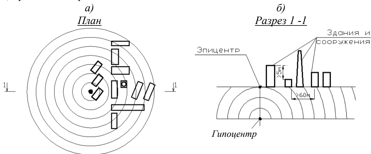
Рис. 24. Принципиальная схема распространения и влияния горизонтальных и вертикальных сейсмических волн, формируемых в гипоцентре землетрясения массива грунта на здания и сооружения, возведенные на поверхности земли:
