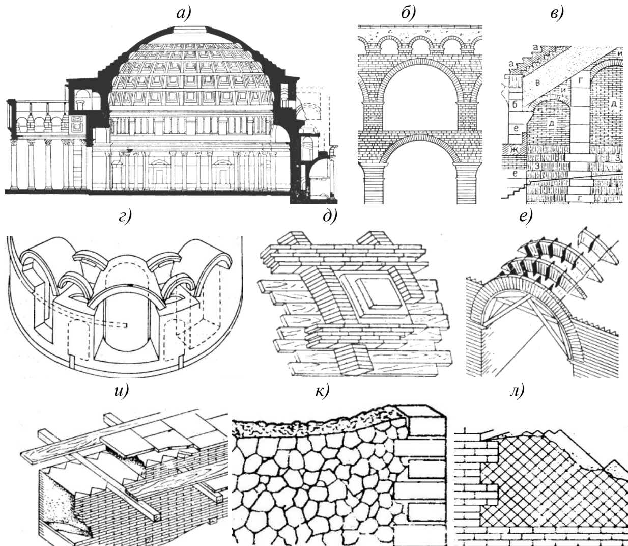
Рис. 8. Сейсмостойкие конструктивные системы древнеримского Пантеона: а-разрез; б-арочная конструкция из каменных квадратов насухо (акведук в Ниме, начало II в.); в-смешанная бетонно-каменная конструкция амфитеатра (Колизей, I в.); г-конструктивная схема ротонды; д, е-технологические схемы возведения кирпично-бетонных сводов; и-бетонная стена с кирпичной облицовкой; к-облицовка стен способом «инцерт» с нерегулярным рисунком фасада; л-то же, способом «ретикулат» с правильной формой фасада
