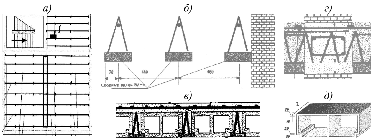
Рис. 37. Конструкции сейсмостойкого междуэтажного перекрытия, состоящего из облегченных мелкоштучных элементов:
