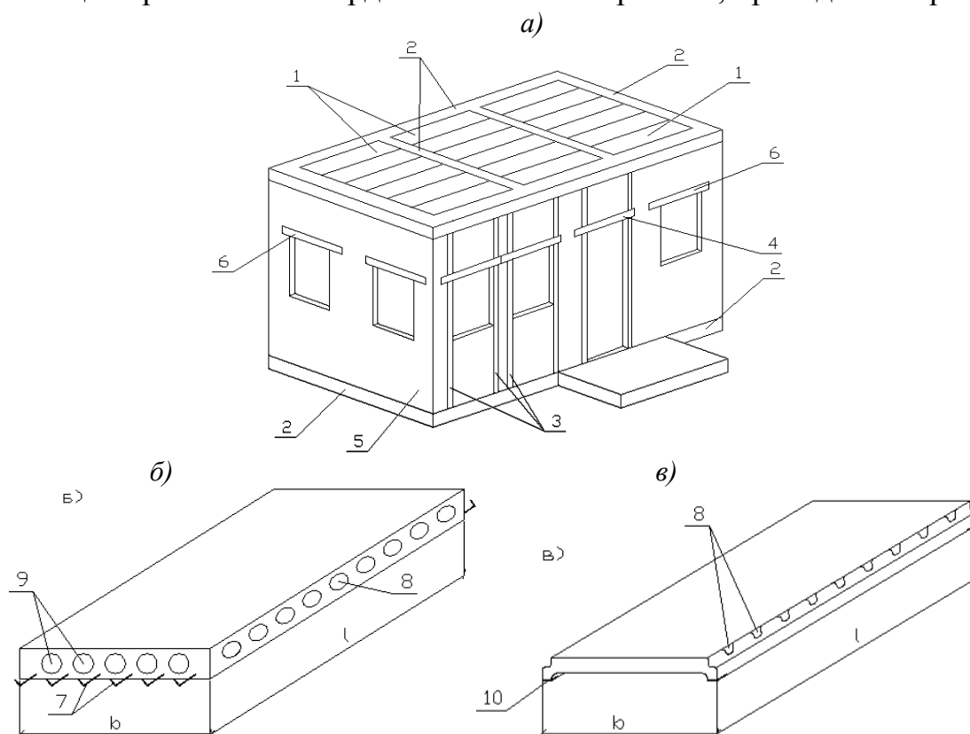
Рис. 71. Принципиальная схема формирования сейсмостойкого здания, возводимого из кирпичной кладки с устройством горизонтального жесткого диска с замоноличиванием сборных железобетонных плит перекрытий в сейсмопояса на уровне перекрытия и элементов упрочнения стен при помощи вертикальных сердечников в зоне проемов: а – схема с элементами замоноличивания и обеспечение жесткости перекрытий и здания в целом; б – аксонометрическая схема сборной ж/б многопустотной плиты перекрытия с арматурными выпусками в торцевых зонах; в – то же, ребристая плита перекрытия с закладными деталями в опорных точках ребер жесткости; 1 – сборные ж/б многопустотные плиты перекрытия; 2 – антисейсмические пояса замоноличивания по типовой серии 2.140-5с, вып.1; 3 – ж/б вертикальные сердечники (монолитные или сборные) в кладке стен по серии 2.130-6с, вып.1; 4 – ж/б перемычки (монолитные или сборные) по серии 2.130-6с, вып.1; 5 – каменные стены; 6 – сборные ж/б перемычки; 7 – арматурные выпуски из сборных ж/б плит для анкерования в монолитный ж/б сейсмопояс; 8 – шпонки на продольной боковой поверхности плиты; 9 – круглые продольные пустоты в плитах перекрытий; 10 – закладные детали для соединения с опорой
