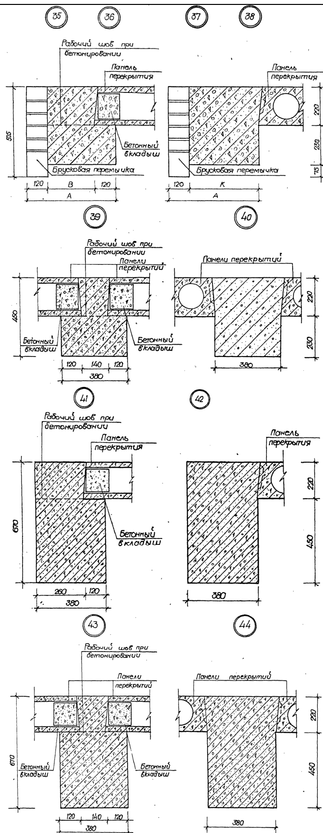
Рис. 7. Узлы №33 - №44. Комплексные конструкции. Примеры сечений поясов перемычек в стенах толщиной 380, 510 и 640 мм, при высоте этажа 2,80 м и 3,00 м
