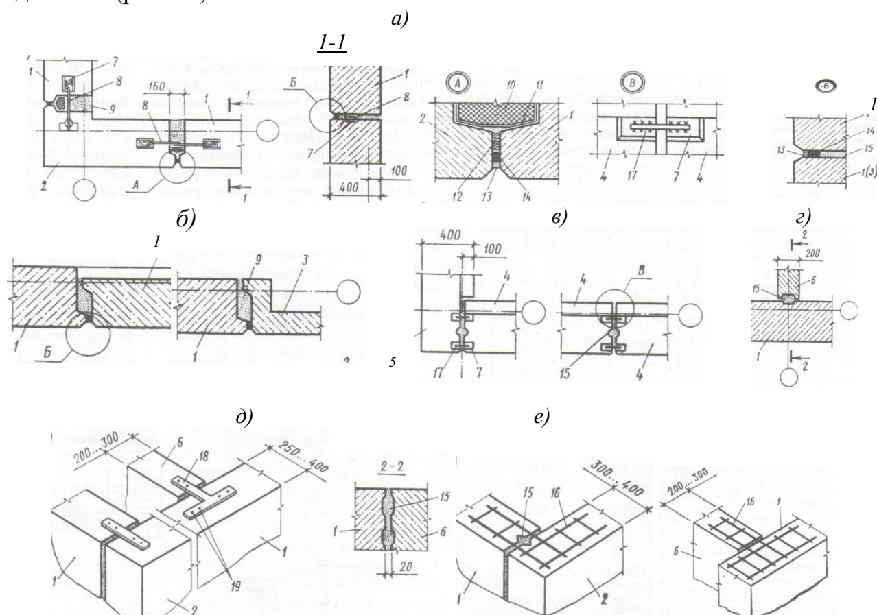
Рис. 69. Узлы сопряжений крупных стеновых блоков наружных стен:
