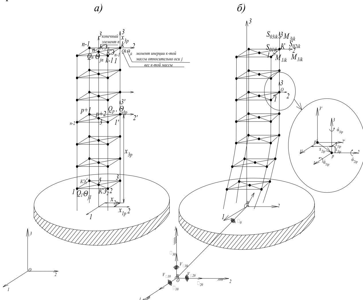
Рис. 20. Пространственная расчетная динамическая модель (РДМ) здания: а - состояние покоя; б - i -я форма колебаний
