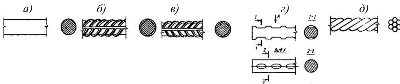
Рис. 51. Арматура для железобетонных конструкций: а-стержневая (класса А-I); б-стержневая (класса А-II); в-стержневая (класса А-III и выше); г-высокопрочная проволока; д-арматурный канат
