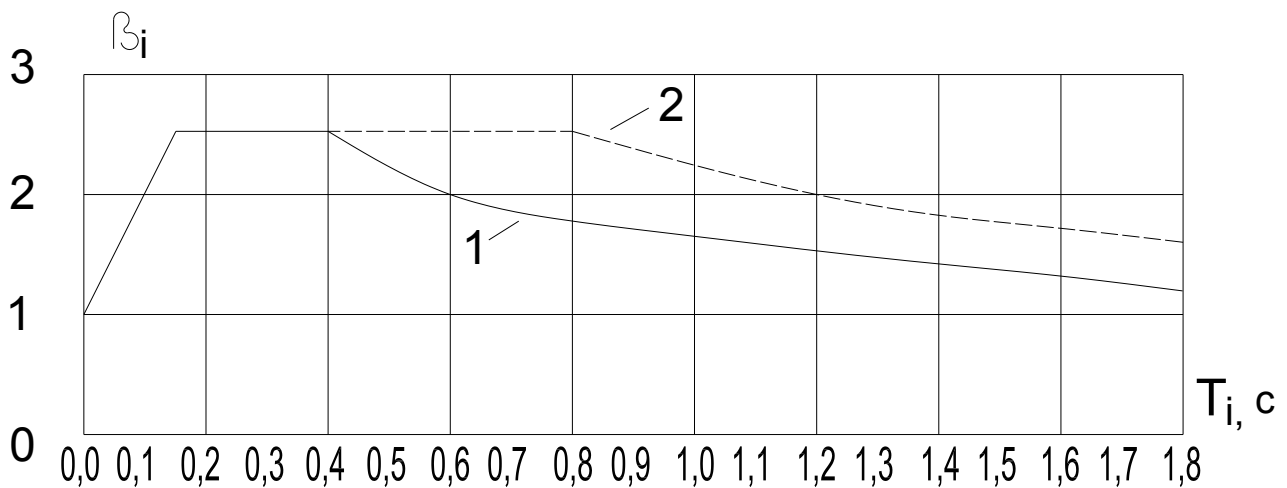
Рис. 22. График зависимости коэффициента динамичности \beta_i от расчётного периода собственных колебаний T_i здания или сооружения по i -ой форме при определении сейсмических нагрузок
