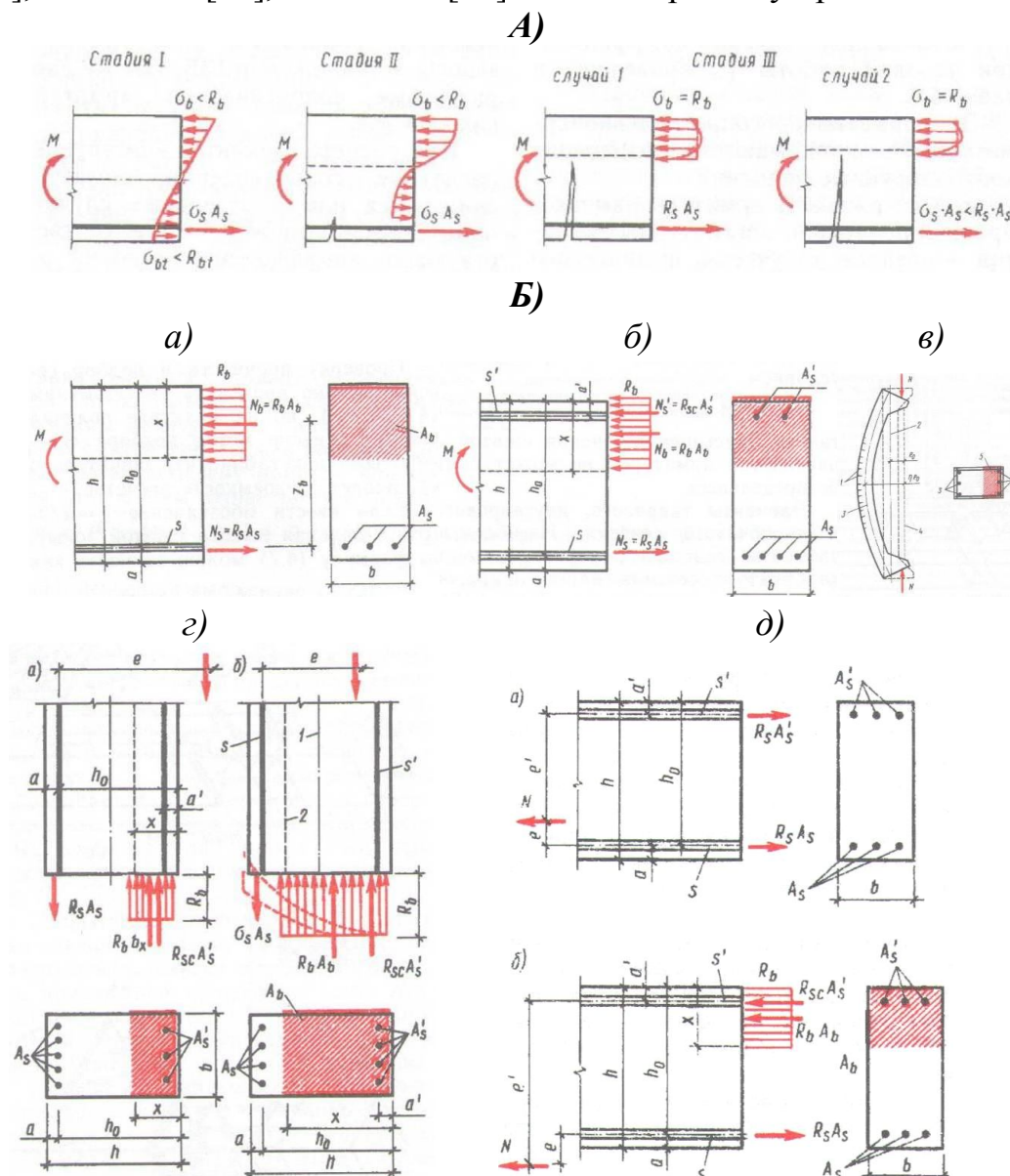
Рис. 50. Схемы к расчету на прочность по нормальному сечению изгибаемых и внецентренно сжатых железобетонных элементов: А -стадии напряженно-деформированного состояния при изгибе (I-упругая стадия; II-появление и раскрытия трещин в бетоне; III-предельная стадия); Б -схемы усилий при расчёте прочности элемента по нормальному сечению: а -с одиночной арматурой; б -то же, с двойной арматурой; в -внецентренно сжатый железобетонный элемент: 1-трещины в растянутой зоне; 2-геометрическая ось элемента до нагружения; 3-то же, после нагружения; 4-ось приложения силы; 5-сжатая зона; г -схема усилий и эпюра напряжений в поперечном сечении внецентренно сжатого элемента: 1-геометрическая ось элемента; 2-граница сжатой зоны; д -то же, внецентренно растянутого элемента
