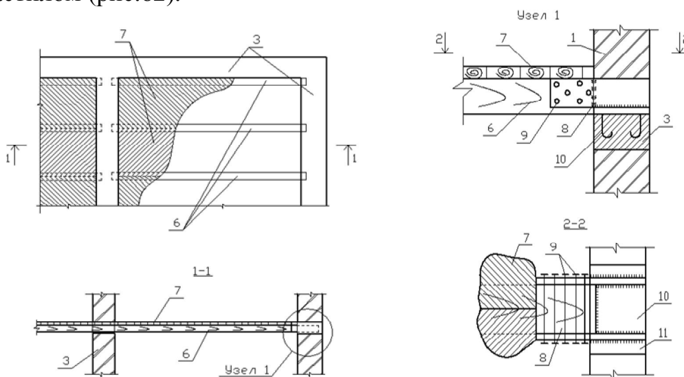
Рис. 82. Конструктивное решение опирания деревянных балок перекрытий и покрытий на кирпичные и каменные стены: 1–кирпичная стена, выполненная на месте строительства, вручную; 3–антисейсмический пояс по типовой серии 2.140-5с, вып.1; 6–деревянные антисептированные балки перекрытия (покрытия); 7–диагональный дощатый настил; 8 –металлический опорный кронштейн; 9 –стяжные болты; 10 – закладная деталь; 11 – сварной шов
