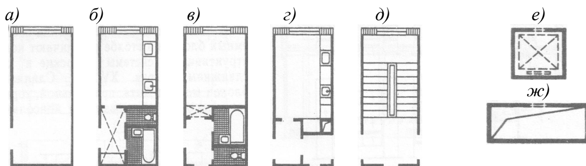
Рис. 63. Типы объемных блоков в зависимости от назначения: а – жилая комната; б – санитарно-кухонный блок; в, г – блоки смешанного назначения; д – блок-лестница; е, ж – вспомогательные блоки (шахты лифтов, шахты коммуникаций, блоки лоджий и т.д.)
