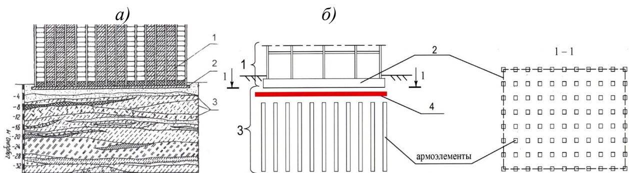
Рис. 33. Плитные конструкции фундаментов под многоэтажные и высотные здания на естественном и искусственно упрочненном грунтовом основании: а -схема разреза по многоэтажному зданию на плитном фундаменте, совмещенному с инженерно-геологическим разрезом, к расчету системы «грунты основания - фундамент - надземное сооружение», где 1-надземное сооружение; 2-плитный фундамент здания; 3-грунтовое основание здания; б -схема сейсмостойкого плитного фундамента многоэтажного здания, возведенного на упрочненном вертикальным армированием грунтовом основании с промежуточной демпфирующей подушкой, рассчитываемом по системе «армированный грунт основания – плитный фундамент – промежуточная подушка - надземное сооружение», где 1-надземное сооружение; 2-плитный фундамент здания; 3-упрочненное вертикальным армированием грунтовое основание здания; 4-промежуточная демпфирующая подушка из песка или щебня
