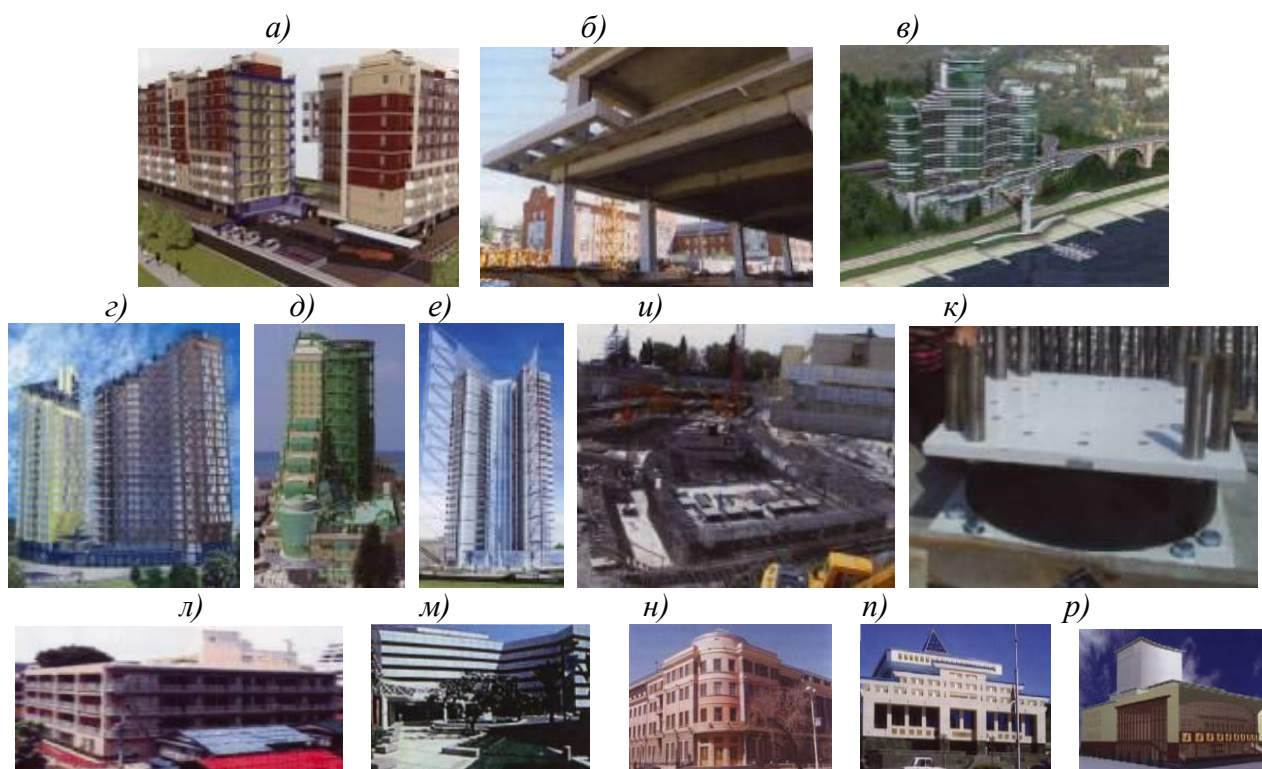
Рис. 15. Здания оборудованные системой сейсмоизоляции и динамического демпфирования: а, б - жилые дома с «гибким» нижним этажом; в –гостиница «Золотая лагуна» в г. Сочи; г, д – высотный жилой дом и деловой центр «Спутник» в г. Сочи; е -гостинично-туристический комплекс «Sea Plaza»; и - возведение сейсмоизолированного фундамента, к - сейсмоизолирующая опора в г. Сочи; л - здание больницы в г. Оджива с сейсмоизолирующим фундаментом; м - Южно-Калифорнийский госпиталь; применение сейсмоизолирующих опор для обеспечения сейсмостойкости реконструируемых зданий, соответственно: н - здание банка в г. Иркутске; п -здание театра в г. Горно-Алтайске; в -концертный зал в г. Грозном
