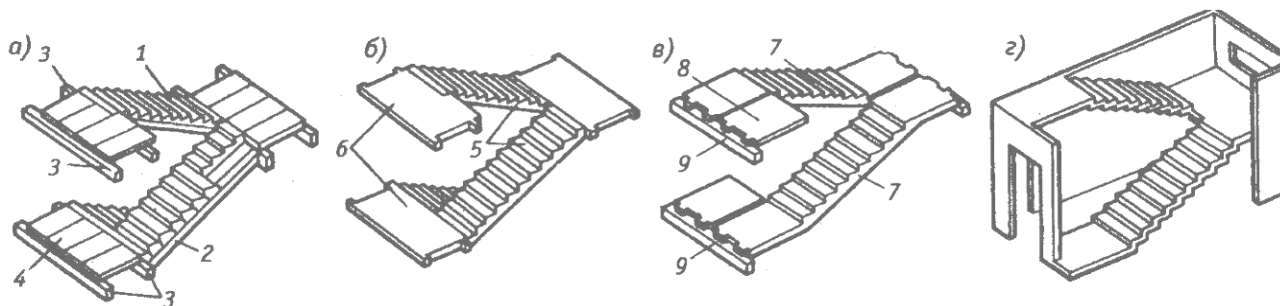
Рис. 39. Конструктивные виды внутренних сборных железобетонных лестниц: а-мелкоэлементная железобетонная лестница на косоурах и балках; б-крупноэлементная лестница, составленная из отдельных лестничных маршей и площадок; в-то же, с маршами, совмещенными с полуплощадками; г-то же, в объемном блоке лестничной клетки; 1-наборные ступени из сборного железобетона; 2-стальные или сборных железобетонные косоуры; 3-то же, балки лестничных площадок; 4-сборные железобетонные мелкоштучные плиты лестничных площадок; 5-лестничные марши; 6-лестничные площадки; 7-лестничные марши с полуплощадками; 8-дополнительная верхняя плита полуплощадки; 9-ригели
