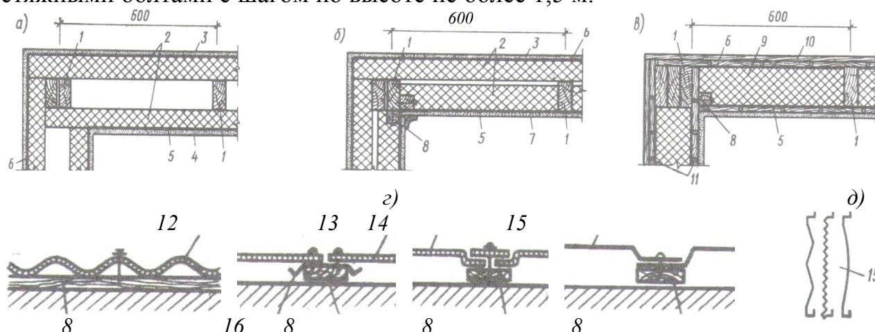
Рис. 74. Примеры заполнения каркасных стен:
