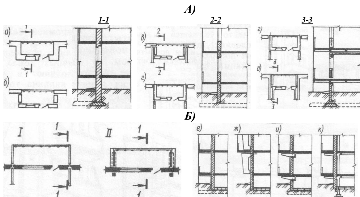
Рис. 48. Конструкции встроенных и выносных лоджий: A) Встроенные лоджии в домах: a -с кирпичными стенами; б -с панельными продольными несущими стенами; в -то же, поперечными несущими стенами; г -то же, с объемным элементом лоджии; д -с объемно-блочными конструкциями; Б) Выносные лоджии в домах: I -панельных; II -каркасно-панельных; е -с несущими стенами лоджий; ж -с навесными стенами лоджий; и -на консолях внутренних несущих стен; к -на консолях колонн каркас
