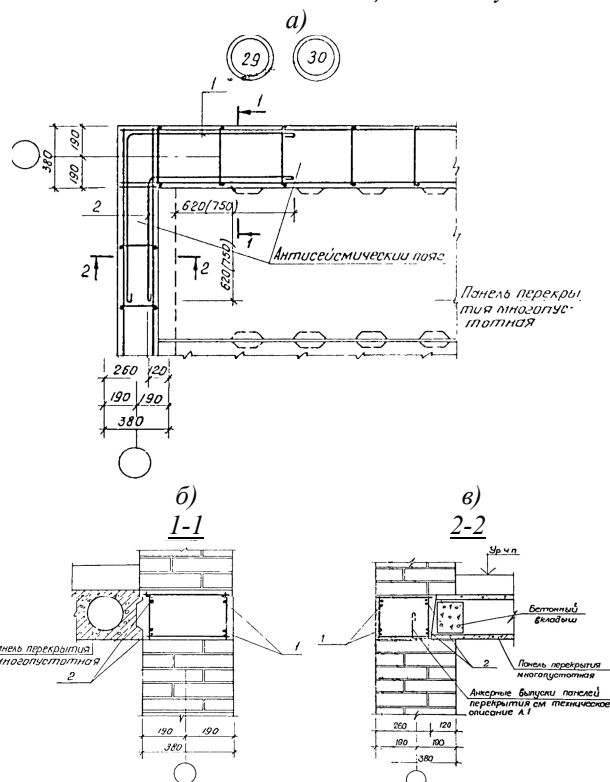
Рис. 9. Узлы № 25, 26, 27, 28 примыкания сборных железобетонных многопустотных панелей перекрытий к внутренним самонесущим кирпичным стенам с вертикальными каналами для вентиляции и дымоудаления
