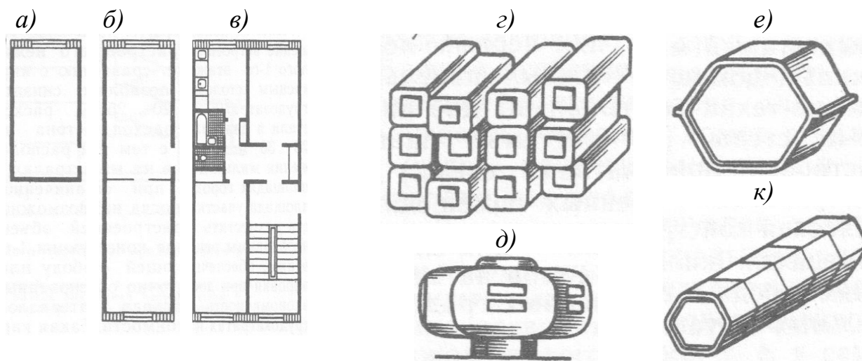
Рис. 64. Типы объемных блоков в зависимости размеров в плане и по форме: а – на комнату; б – на группу помещений; в – на квартиру (включая лестницу); г – прямоугольные; д – криволинейные; е, к – косоугольные
