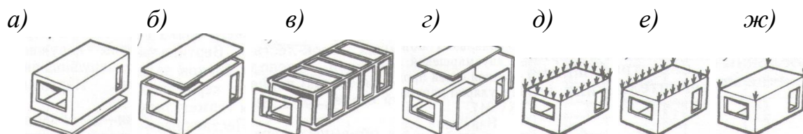
Рис. 65. Типы объемных блоков в зависимости от способов изготовления и условий опирания конструктивных элементов:
