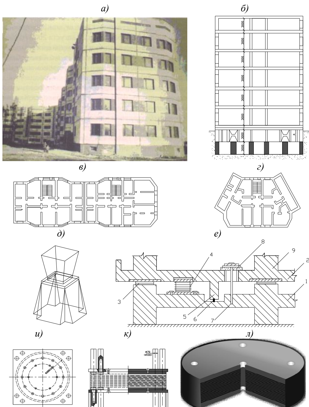
Рис. 1. Сейсмоизоляция существующих зданий и сооружений путем поэтапной установки резинометаллических подушек
