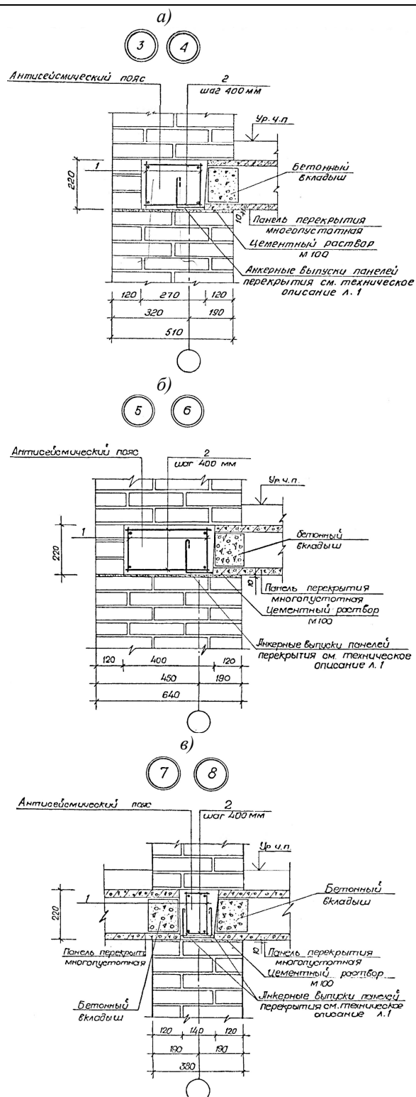
Рис. 3. Узлы опирания сборных многопустотных панелей перекрытий на наружные и внутренние кирпичные стены: а - наружные толщиной 510мм, где узел №3- для 7, 8 баллов, узел №4-для 9 баллов; б - наружные толщиной 640мм, где узел №5-для 7, 8 баллов, узел №6- для 9 баллов; в - внутренние толщиной 380мм, где узел №7-для 7, 8 баллов, узел №8-для 9 баллов
