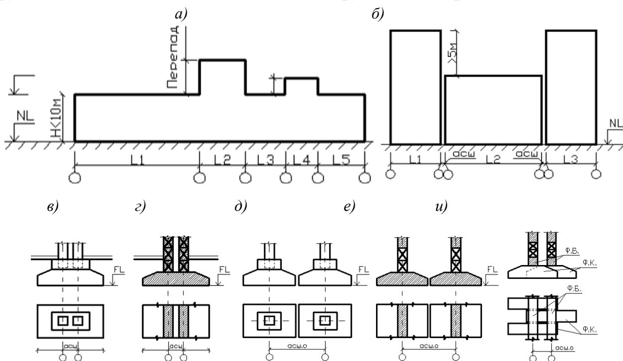
Рис. 26. Антисейсмические швы ( асш , асш.о ) и варианты их устройства: а - схема перепадов для одноэтажных зданий при расчетной сейсмичности 7 баллов; б - схема устройства антисейсмических швов в зданиях с перепадами высот; в - антисейсмический шов ( асш ), не совпадающий с осадочным для зданий с каркасным остовом; г - то же для зданий со стеновым остовом из кирпичных, панельных, блочных и др. конструкций с ленточными фундаментами; д - антисейсмический шов, совпадающий с осадочным для зданий с каркасным остовом; е - то же для зданий со стеновым остовом из кирпичных, панельных, блочных и др. конструкций на сплошных ленточных фундаментах; и - то же для зданий со стеновым остовом на прерывистых ленточных фундаментах (ФК) с фундаментными балками (БФ)
