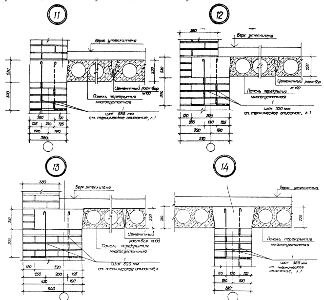
Рис. 5. Узлы анкеровки антисейсмического пояса верхнего этажа при примыкании панелей перекрытий к наружным (№11, №12, №13) и внутренним (№14) стенам толщиной: 380мм для узла №11; 510мм для узла №12; 640мм для узла №13; 380мм для узла №14
