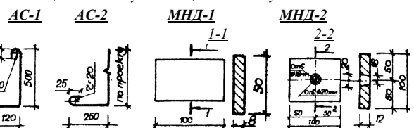
Рис. 6. Чертежи анкерных стержней АС-1 и АС-2 и металлических накладных деталей МНД-1 и МНД-2
