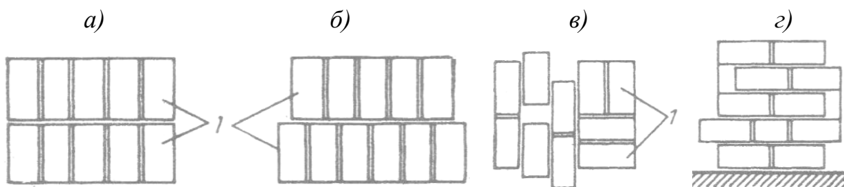
Рис. 62. Схемы зданий из объемных блоков в столбе: а – плоская в плане; б – со сдвижкой в плане по продольной оси; в – со сдвижкой в плане по двум осям; г – со сдвижкой по вертикали; 1 – объемные блоки
