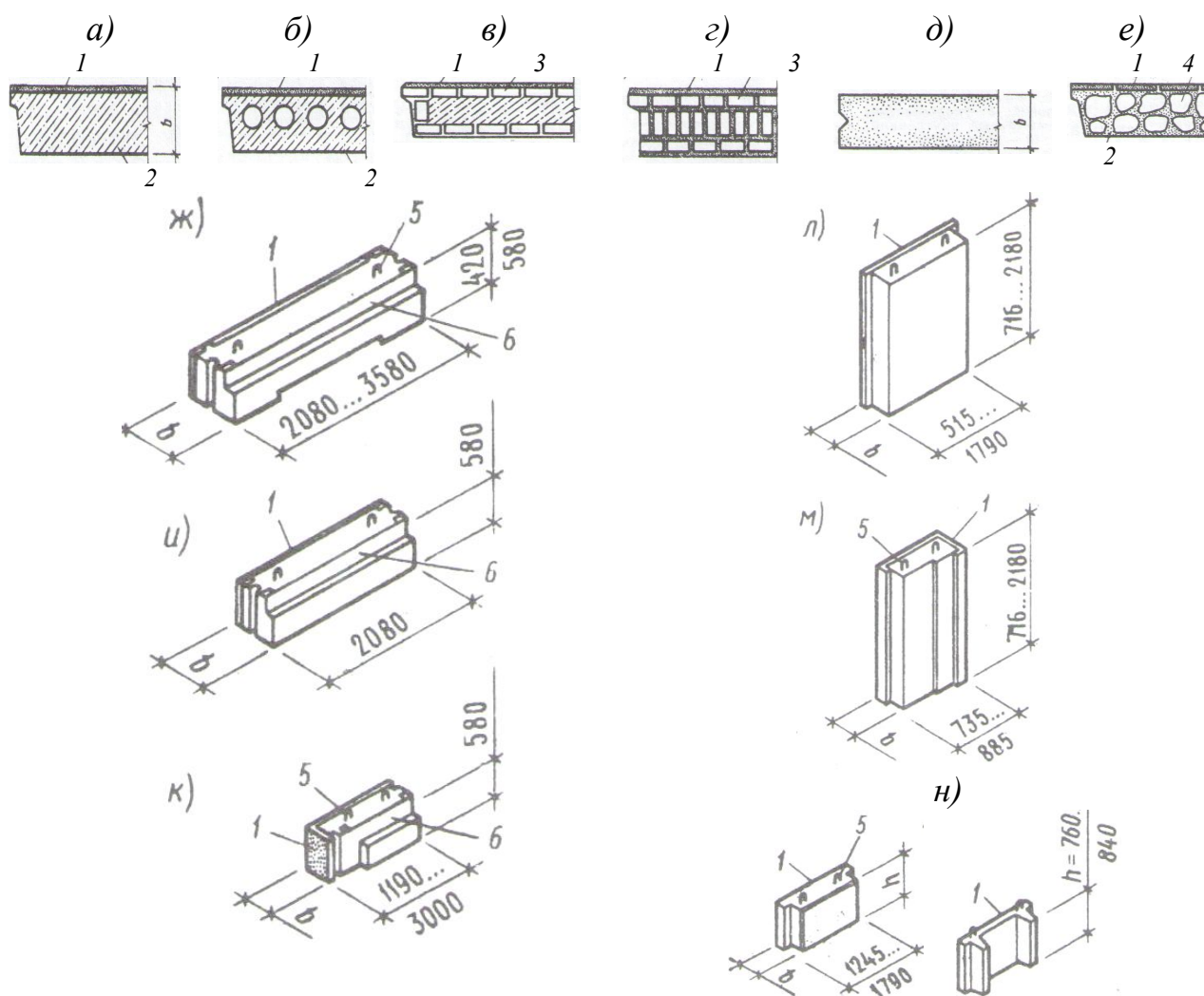
Рис. 68. Конструкции крупных блоков для наружных стен зданий и сооружений: а... е - конструкции крупных блоков; ж... и - габаритные схемы, в том числе: а - сплошной лег- кобетонный; б - с пустотами; в - кирпичный с легкобетонным вкладышем; г - из эффективно- го кирпича; д - из природного камня или арболита; е - из природного камня на легкобетонной связке; ж - перемычный крупный стеновой блок; и - поясной (рядовой); к - поясной угло- вой; л - простеночный рядовой; м - простеночный угловой; н - подоконные блоки; 1 - фасадная сторона (фактурный слой); 2 - легкий бетон; 3 - кирпич; 4 - природный камень ма- лой плотности ( \rho < 1600 \text{ кг/м}^3 или удельным весом \gamma < 16,00 \text{ кН/м}^3 ); 5 - монтажная петля; 6 - полка для опоры элементов перекрытия
