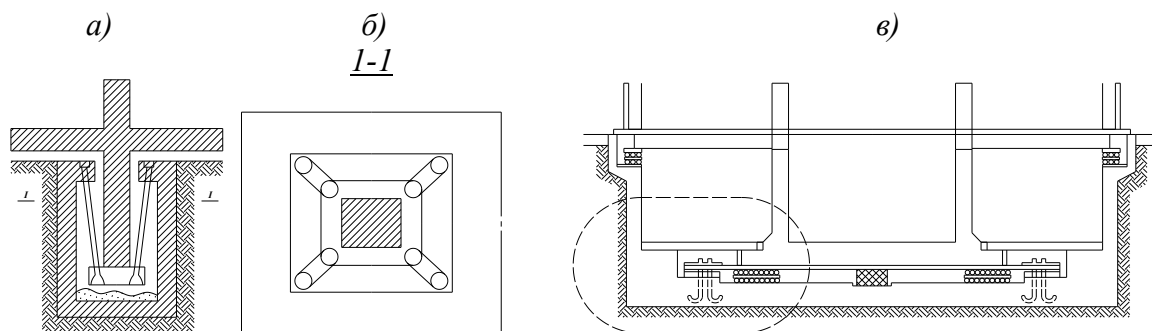
Рис. 14. Маятниковый (а, б) и комбинированный (в) способы сейсмоизоляции зданий и сооружений: а - поперечный разрез фундамента с подвеской на четырех тросах; б - сечение I-I по конструкции маятниковой сейсмоизоляции; в - система комбинированной (комплексной) сейсмоизоляции здания, возведенного на фундаменте глубокого заложения (ФГЗ)
