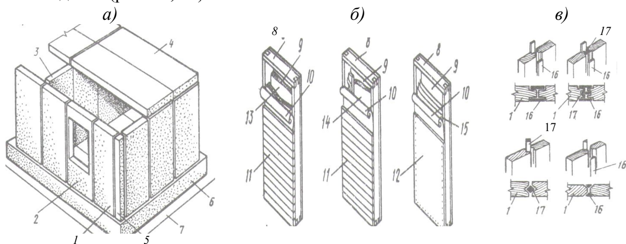
Рис. 78. Панельное щитовое здание с основными деталями и узлами:
