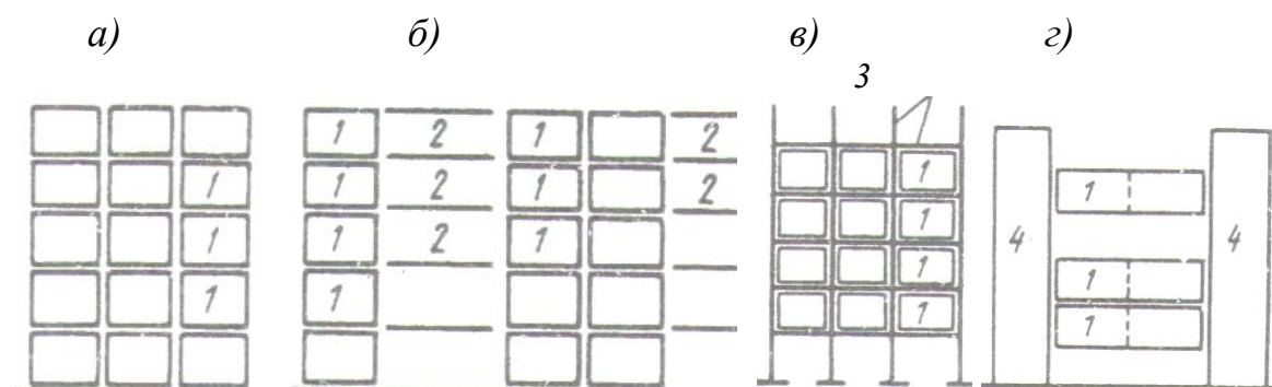
Рис. 61. Конструктивные схемы зданий с применением объемных блоков: а - «чисто» блочная; б - панельно-блочная; в - каркасно-блочная; г - блочно-ствольная; 1 – объемные блоки; 2 – панели перекрытия; 3 – каркас; 4 – ядра жесткости (стволы)
