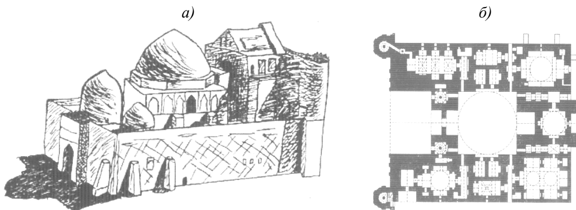
Рис. 9. Сооружение мавзолея Ахмеда Ясави: а-общий вид, б-план мавзолея с разделением на восемь независимых объемных блоков осадочными швами
