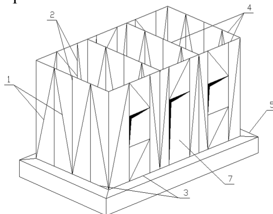
Рис. 81. Принципиальная схема пространственного деревянного каркаса, заполняемого местным строительным материалом: 1 –диагональные связи; 2 –вертикальные стойки на врубках; 3 –нижние замкнутые брусья-лежни; 4 –верхние замкнутые брусья-поояса; 5 –ленточный фундамент; 6 –оконный проем; 7 –дверной проем
