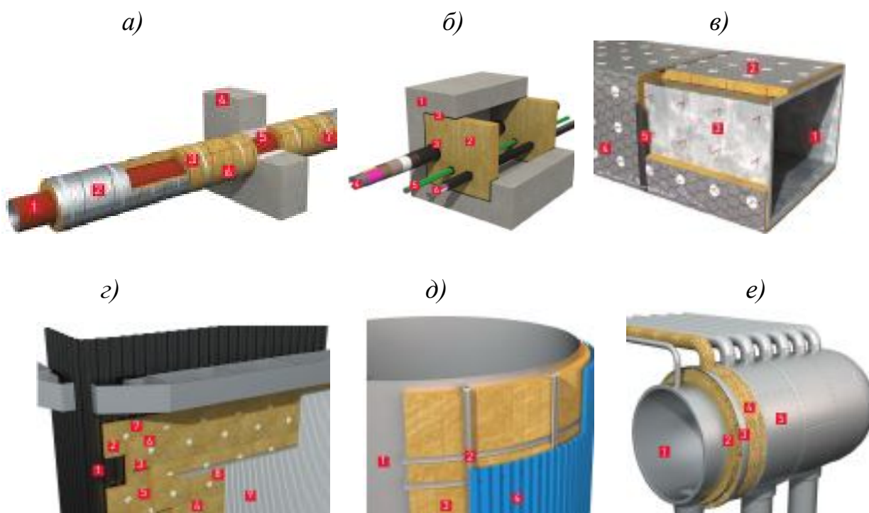
Рис. 89. Принципиальные конструктивные решения по огнетеплозащите инженерных систем коммуникаций и оборудования зданий или сооружений:
