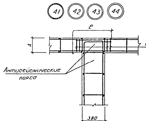
Рис. 13. Узлы № 35, 36, 37, 38, 39, 40 сопряжения антисейсмических поясов в плане
