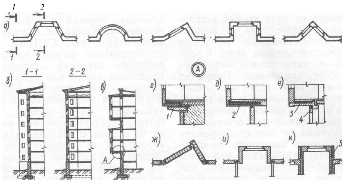
Рис. 49. Конструкции эркерov: a -формы планов эркерov; б -эркер с несущими стенами; в -навесной эркер; г -навесной эркер в панельном доме, опертый на консоли внутренних стен; д -то же, на утепленную консоль перекрытия; е -то же, в кирпичном доме, эркер оперт на консольную керамзитобетонную плиту; ж -стены эркерov из панелей; и -то же, из объемного элемента; к -устройство эркера в объемно-блочном доме; 1 -железобетонная консоль панели внутренней стены; 2 -консоль перекрытия; 3 -консольная керамзитобетонная плита эркера; 4 -оконная перемычка; 5 -утепляющая панель
