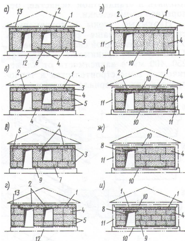
Рис. 67. Схемы разрезки стен одноэтажных жилых зданий на крупные стеновые блоки:
