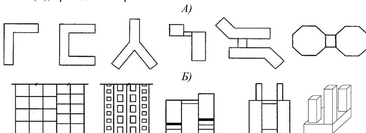
Рис. 19. Схемы зданий со сложными конструктивно-планировочными решениями:
