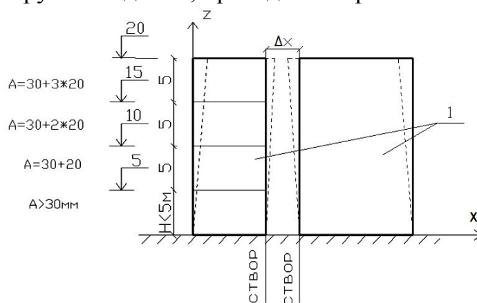
Рис. 27. Схема к назначению расчетной ширины антисейсмического шва \Delta x «в свету», между створами примыкающих конструктивных элементов блокируемых зданий: 1 –отсеки примыкающих блоков здания или сооружения
