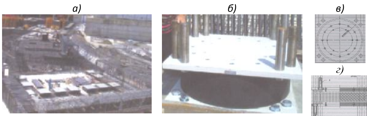
Рис. 86. Возведение сейсмоизолированного фундамента с применением сейсмоизолирующих резинометаллических опор на объекте «Гостинично-туристический комплекс «Sea Plaza» в г. Сочи: а-возведение сейсмоизолированного фундамента; б-общий вид сейсмоизолирующей резинометаллической опоры перед возведением надземной части здания; в, г-схема плана и разреза конструкции резинометаллической опоры
