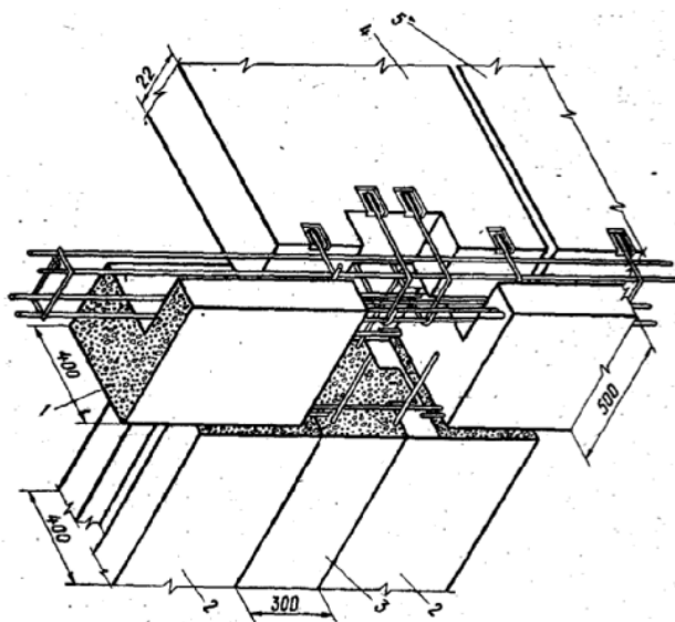
Рис. 70. Аксонометрический узел сопряжения элементов сейсмостойкого сборного железобетонного каркаса с крупными блоками каркасно-блочного здания: 1-перемычный блок; 2-простеночный блок; 3-железобетонная колонна; 4-сборная железобетонная межколонная панель перекрытия; 5-сборная железобетонная многопустотная рядовая панель перекрытия
