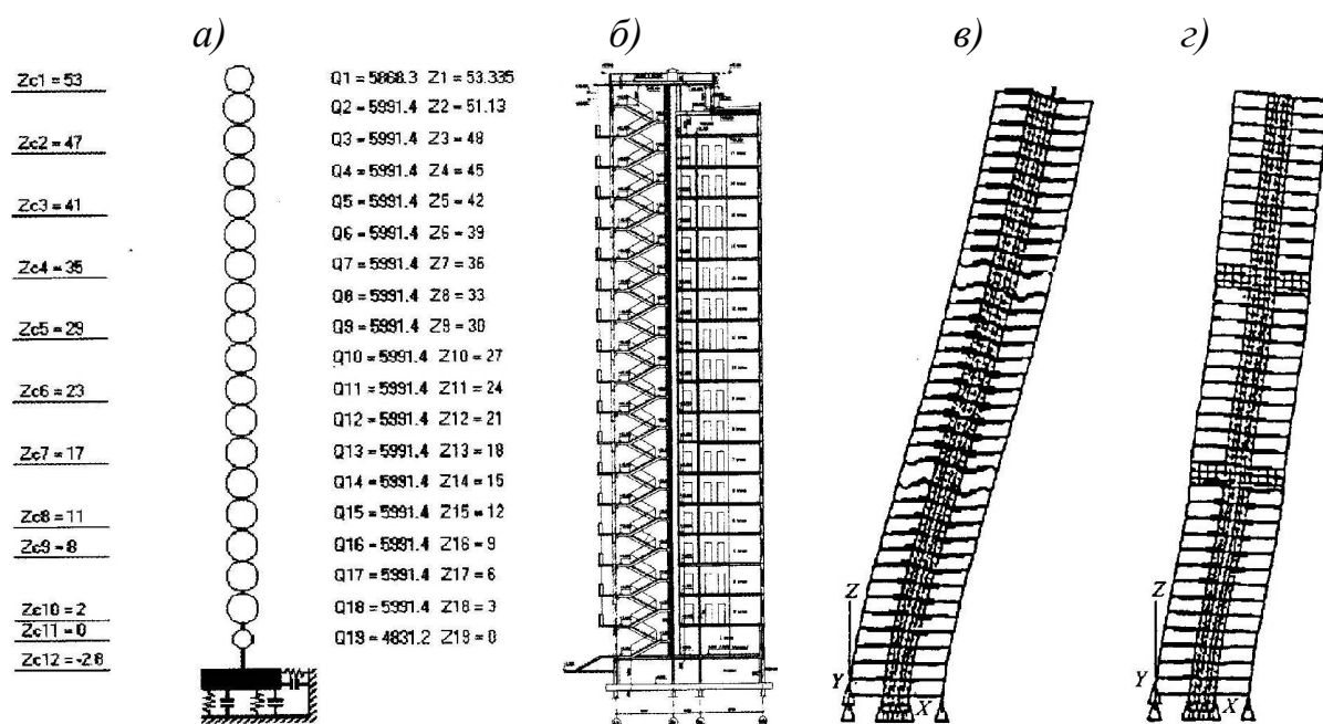
Рис. 84. Сейсмоизоляция и сейсмозащита высотных зданий: а-схема к расчету здания с демпфирующими системами на сейсмические воздействия; б-поперечный разрез сейсмостойкого высотного здания; в-деформации здания, возведенного без усиленных этажей; г-то же, с жесткими этажами
