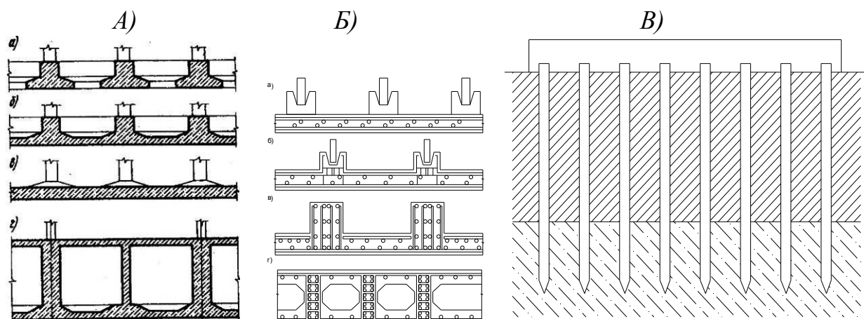
Рис. 32. Типы фундаментов многоэтажных зданий и сооружений, возводимых на нескольких дисперсных грунтах в сейсмически активных районах:
