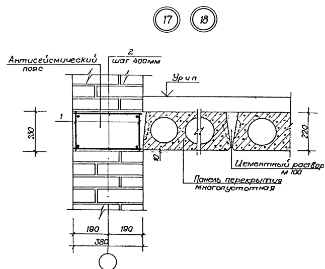
Рис. 7. Узлы № 17, 18 для наружных стен толщиной 380мм примыкания сборных многпустотных панелей перекрытий к наружным и внутренним самонесущим кирпичным стенам, где узел №17-для 7, 8 баллов, узел №18-для 9 баллов
