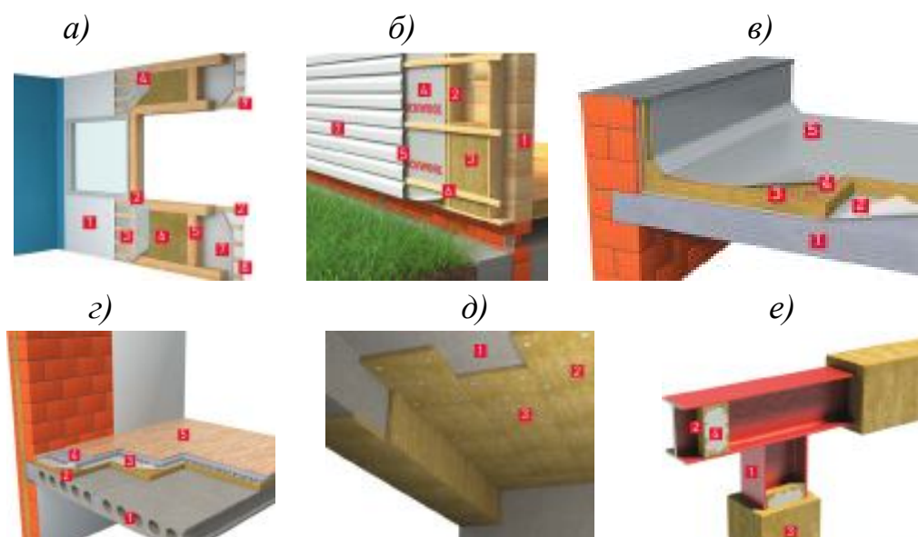
Рис. 88. Принципиальные конструктивные решения по огнетеплозащите несущих и ограждающих конструкций остовов зданий или сооружений:
