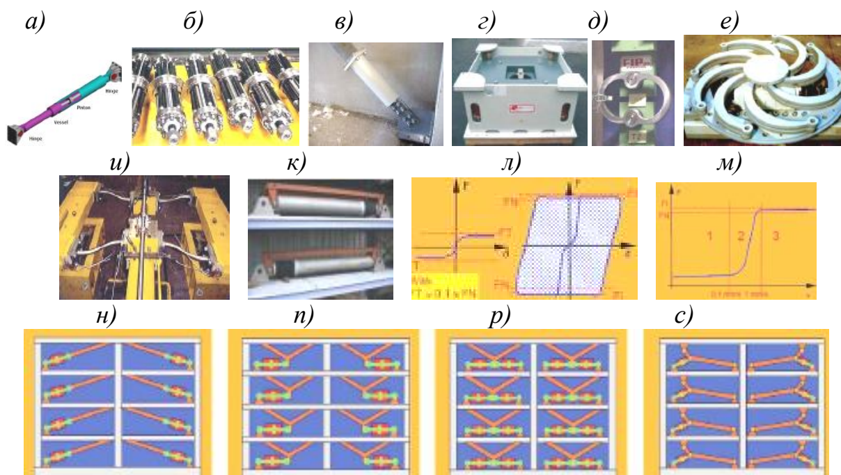
Рис. 85. Современные системы разработанных отечественными и зарубежными учеными и специалистами демпфирующих элементов, получивших наибольшее распространение в мировой практике:
