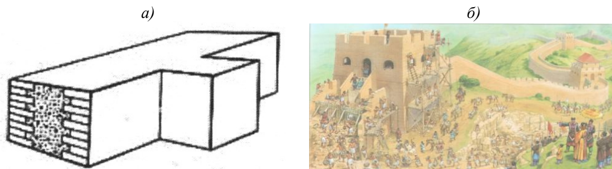
Рис. 5. Сейсмостойкие конструкции древней многослойной кладки стен: а -фрагмент древней многослойной массивной кладки с контрфорсом, состоящей из среднего податливого слоя, выполненного из кладки сырцового кирпича на глиняном растворе и облицованной с двух сторон слоями из кладки обожженным (керамическим) кирпичом; б -Великая Китайская стена с технологическими приемами строительных процессов
