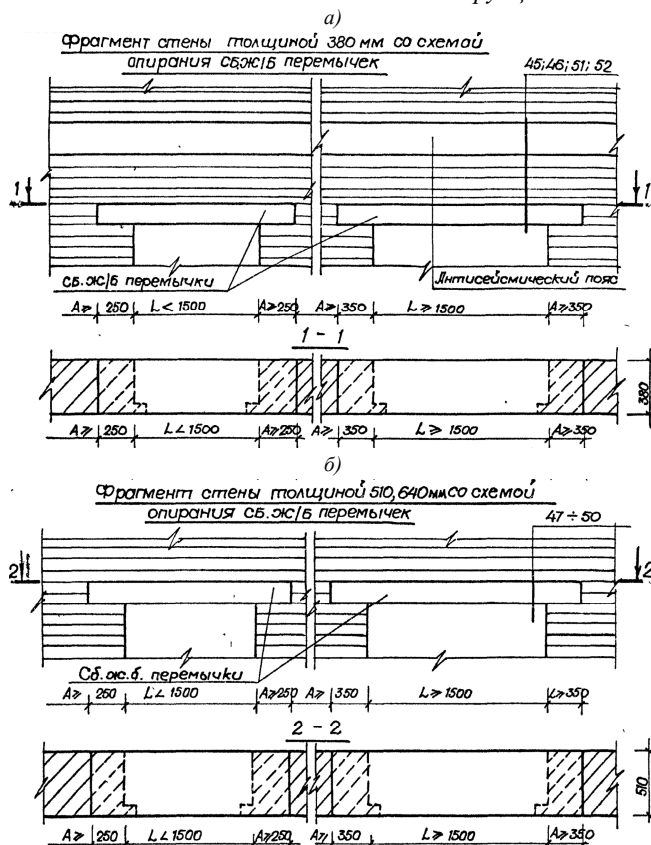
Рис. 4. Конструктивные решения фрагментов кирпичных стен толщиной 380 мм, 510 мм и 640 мм с проемами в сейсмически активных районах: а – фронтальная проекция и сечение 1-1 (горизонтальная проекция) фрагмента стены толщиной 380 мм со схемой опирания сборных железобетонных перемычек на кирпичные простенки (при ширине проема L < 1500 мм (схема слева) и L \geq 1500 мм (схема справа) без учета четвертей в кладке, минимальная длина опирания «А» перемычки на кирпичную кладку простенка с каждой стороны, должна быть, соответственно, не менее A \geq 250 мм (схема слева) и A \geq 350 мм (схема справа), или при L < 1500 мм, A \geq 250 мм, а при L \geq 1500 мм, A \geq 350 мм); б – то же, для стен толщиной 510 мм и 640 мм
