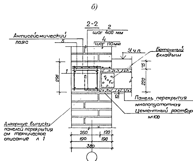
Рис. 5. Узлы № 13, 14, 15, 16 опирания сборных многослойных панелей перекрытий на крайние несущие кирпичные стены с вертикальными каналами для вентиляции и дымоудаления. а – фрагмент плана и разрез 1-1; б – сечение 2-2 к узлам № 13, 14, 15, 16
