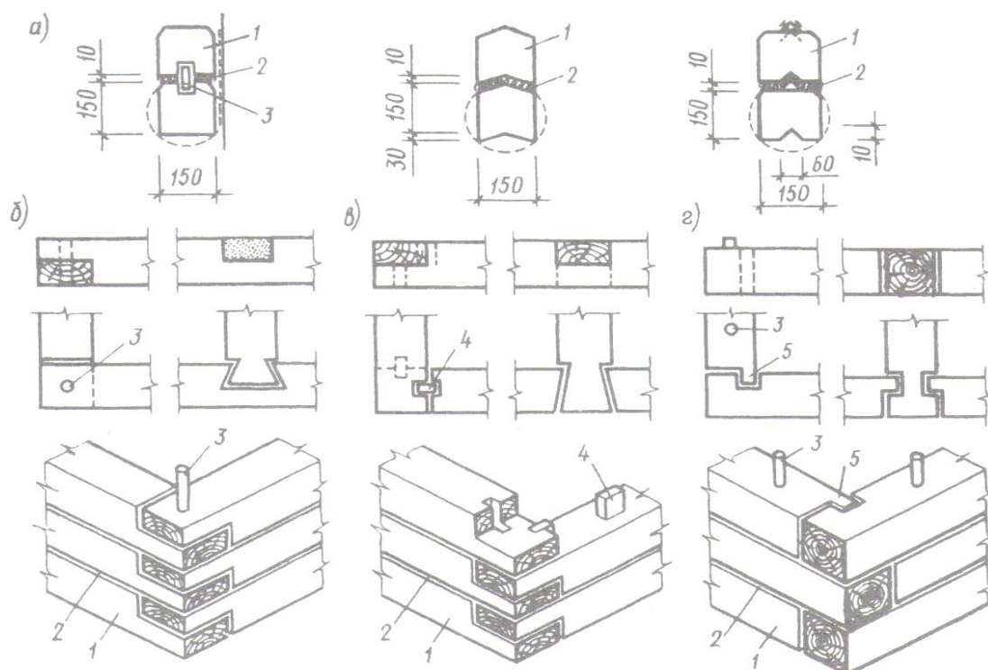
Рис. 76. Узлы и детали брусчатых деревянных конструкций стен: а -сечения брусчатых стен; б, в, г –сопряжения брусьев в углу и с внутренней стеной; 1 –брус; 2 –конопатка; 3 –нагель; 4 –шип; 5 –коренной шип
