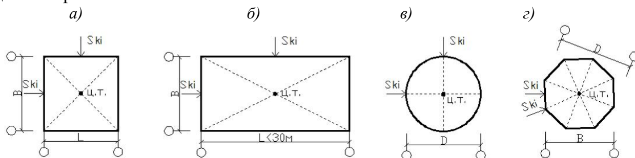
Рис. 16. Простейшие симметричные геометрические формы схем зданий в плане с векторами приложения сейсмических сил S_{ki} , совпадающими с главными центральными осями, проходящими через центр тяжести (ц.т.) фигуры: а - квадратная; б - прямоугольная; в - круглая; г - многоугольная
