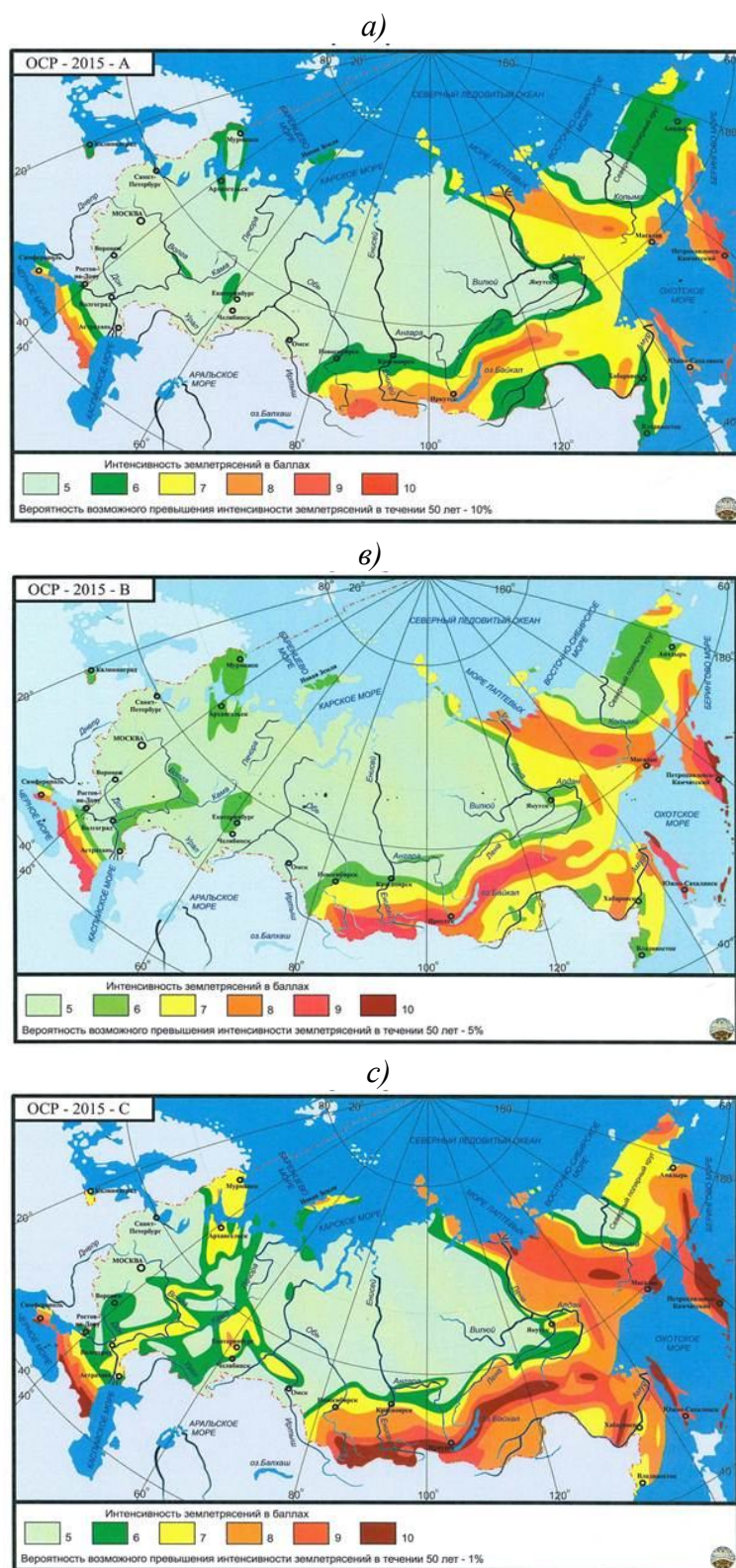
Рис. 17. Комплект карт общего сейсмического районирования территории Российской Федерации (ОСР-2015): а - вероятность возможного превышения интенсивности землетрясений в течение 50 лет -10%; в -то же, 5%; с - то же, 1%
