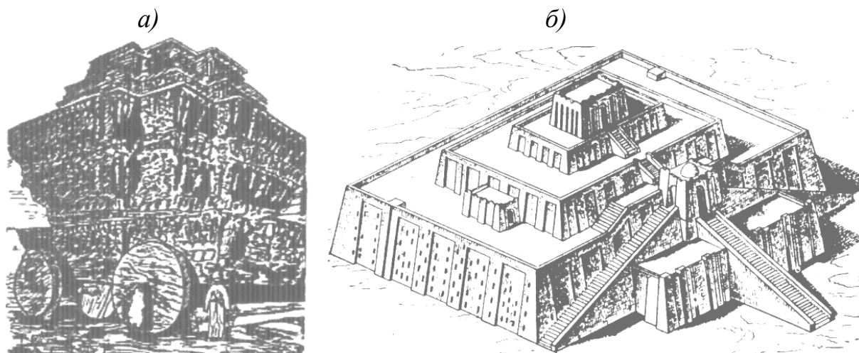
Рис. 6. Примеры древних сейсмостойких монументальных сооружений: а - древний индийский храм на платформе с колесами; б - Зиккурат в Уре, конец III века д н.э. высотой 15 м над поверхностью земли, покоящийся на платформе 43х65 м
