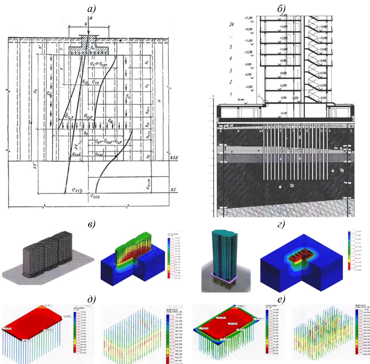
Рис. 35. Основные расчетно-конструктивные схемы распределения напряжений в армированном массиве по результатам инженерных расчетов и расчетов методами конечных элементов при помощи программного комплекса «Midas»: а- расчетная схема развития напряжений в массиве просадочного грунта, армированного вертикальными армозементами (модель автора настоящего издания); б-инженерно-геологический разрез, совмещенный с разрезом многоэтажного здания на плитном фундаменте, возведенном на армированном грунтовом основании; в-расчетная модель и вертикальные деформации для многоэтажного здания на плитном фундаменте; г-расчетная модель и вертикальные деформации для многоэтажного здания на плитном фундаменте; д-вертикальные деформации и усилия в свайных элементах; е-вертикальные деформации и усилия в армирующих элементах
