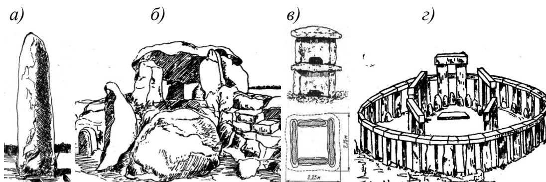
Рис. 4. Мегалитические сооружения эпохи первобытно-общинного строя: а -менгир; б -дольмен эпохи позднего неолита; в -двухэтажный сейсмостойкий дольмен, расположенный вблизи селения Горикди в Азербайджане; г -кромлех в Стронхендже (Англия) с кругом диаметром 30 м
